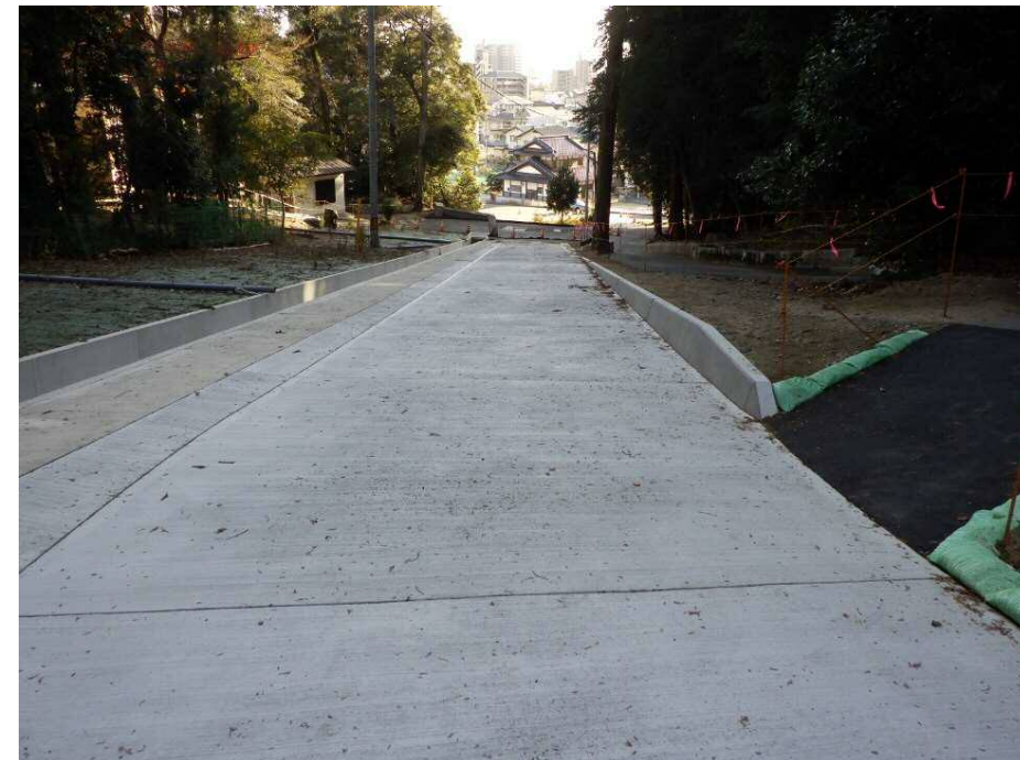
【 施工状況（管理用道路：コンクリート舗装） 】
