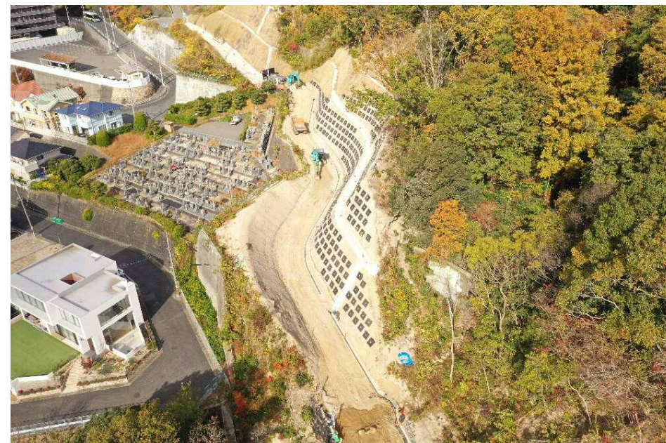
【 施工箇所状況】
