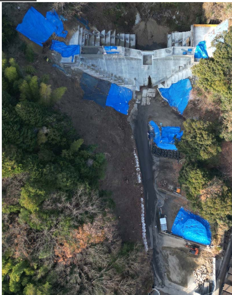
【施工状況（上空より）】
