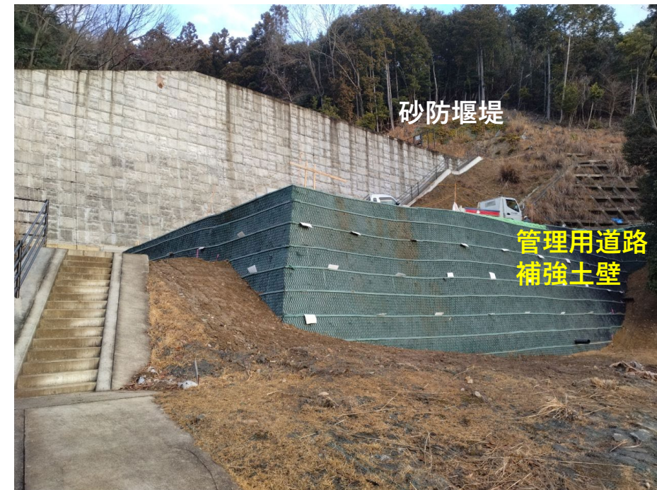
【管理用道路（補強土壁）の施工状況】
