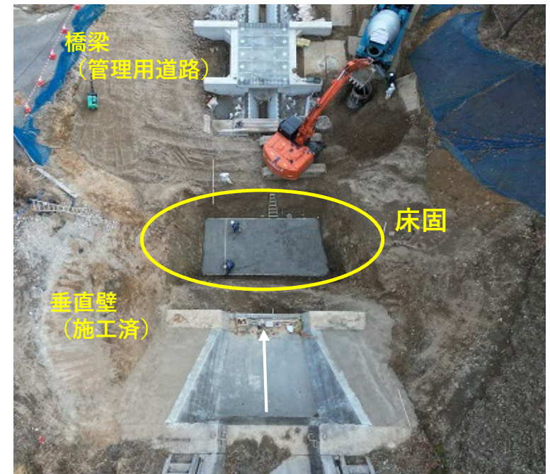
【流路 (床固) の施工状況】
