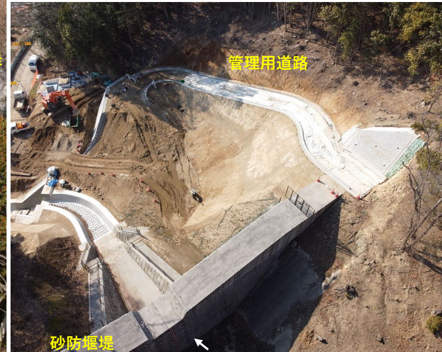
【管理用道路 施工状況】
