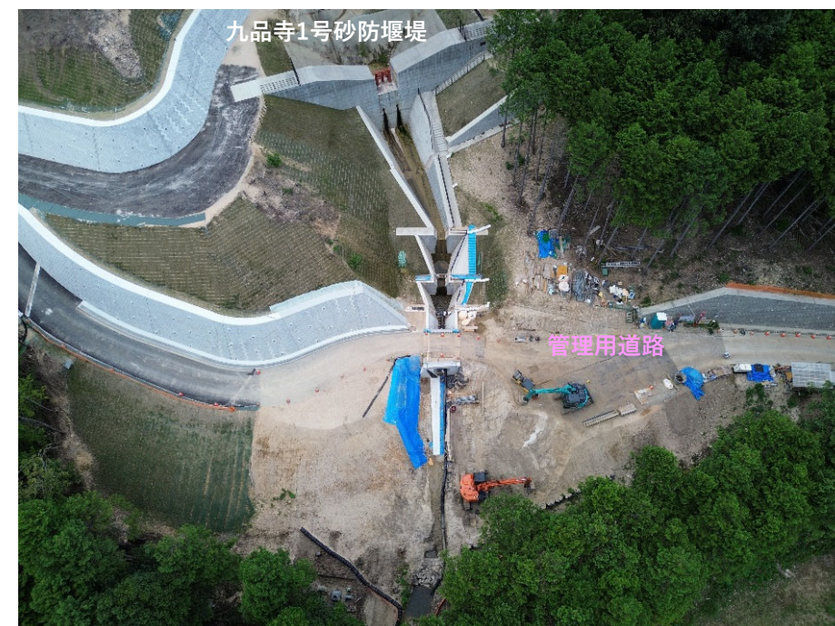
【九品寺1号砂防堰堤溪流保全工箇所 施工状況】
