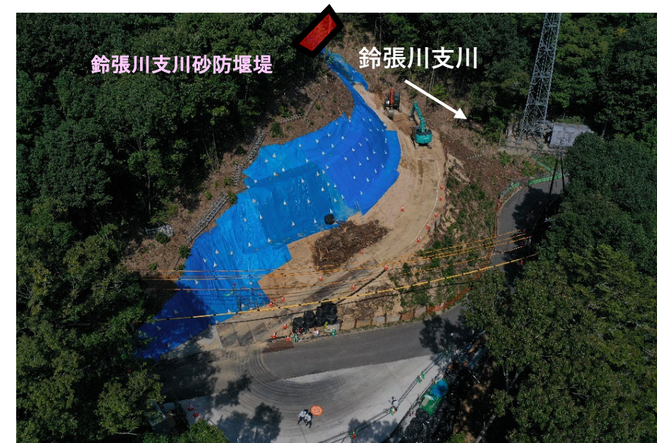
【掘削作業 施工状況】
