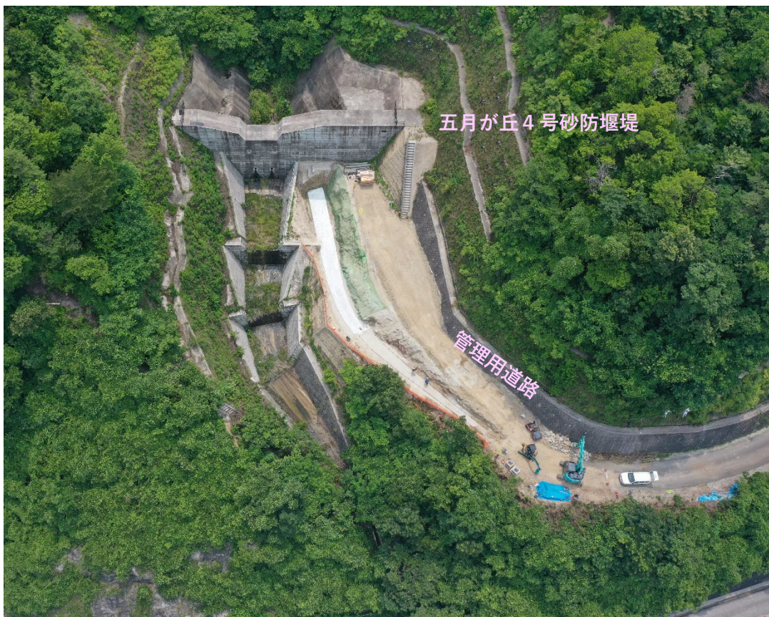
【五月が丘4号砂防堰堤 施工状況】
