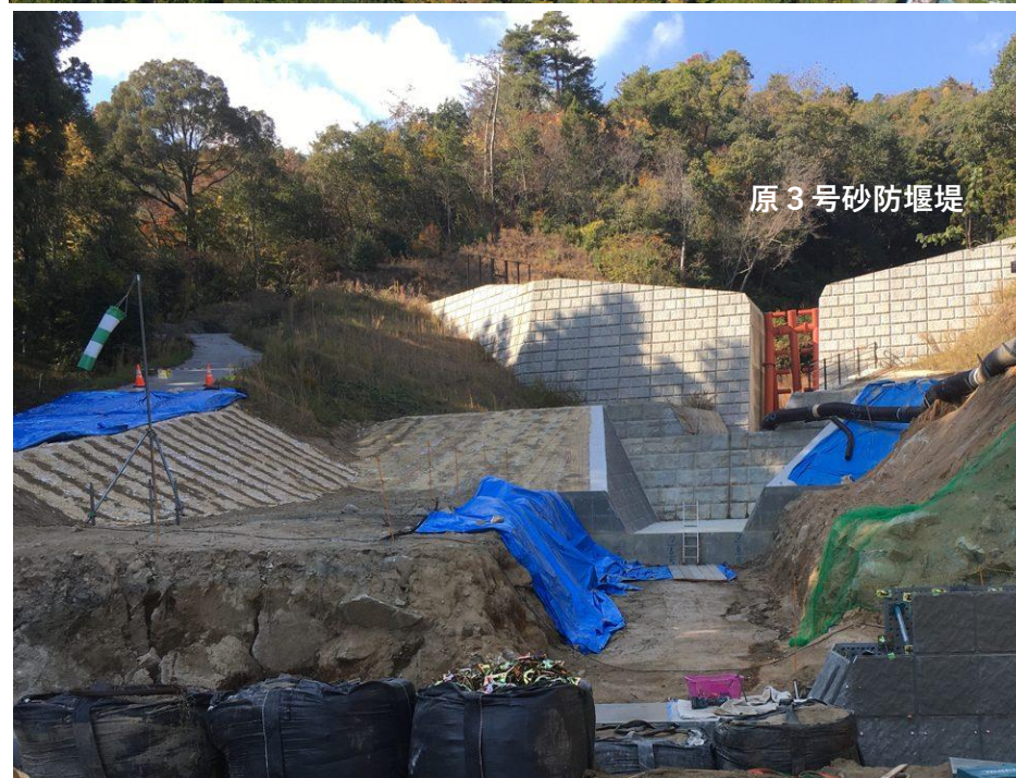
【原3号砂防堰堤下流施工状況】
