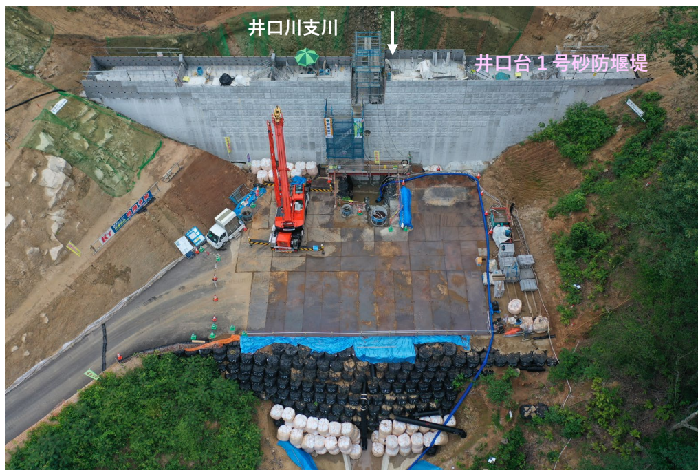
【上空より（堰堤下流から）】
