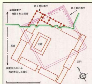
第1期の郡庁(復元想像図)
