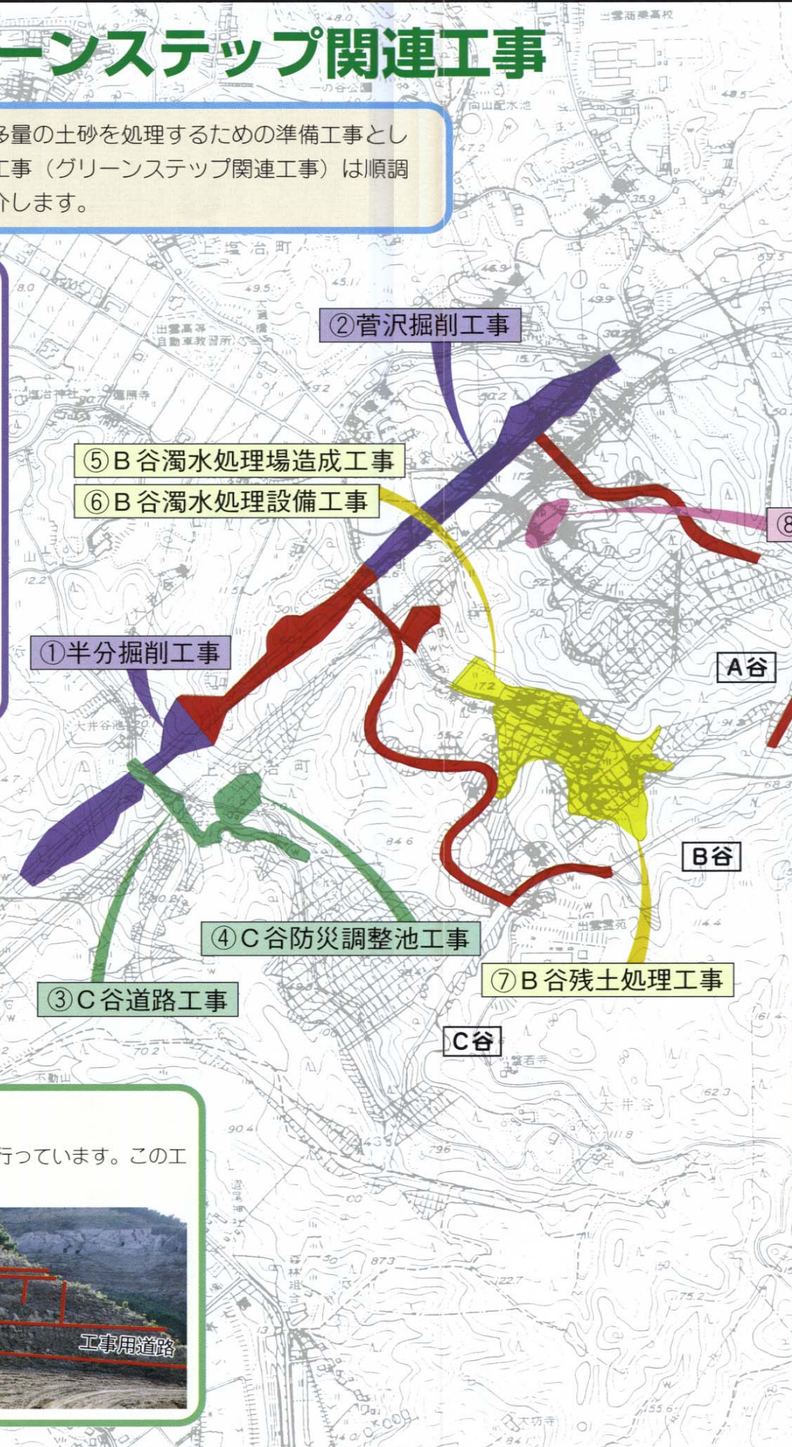
半分掘削工事
