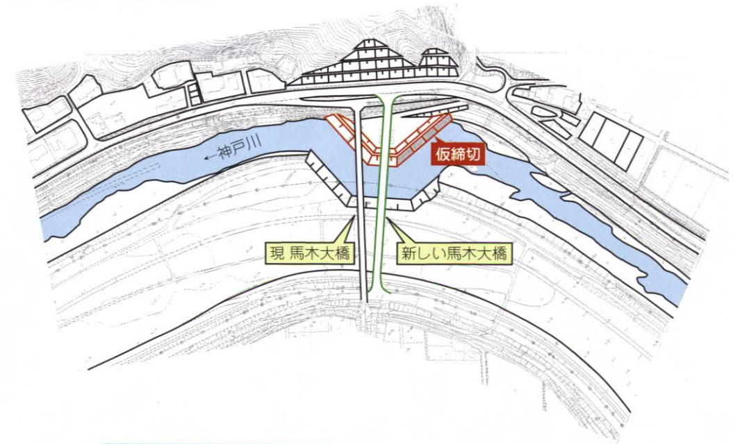
※太破線部が瀬替え前の神戸川河床部です。
