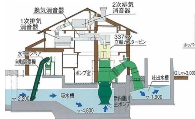
排水機場断面図(新内藤川主ポンプ)
