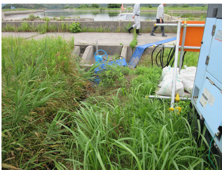
○樋門・仮設排水ポンプ①（道路側より）
