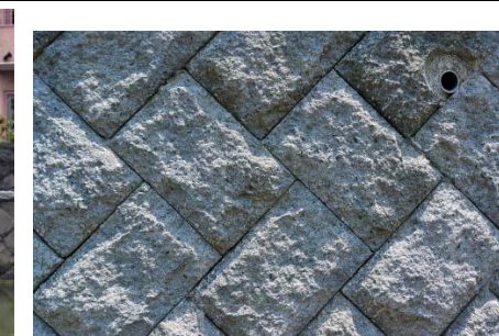
■レベル1-2：表面はつり出しブロック 人工的な面取り部をはつり落とした製品
