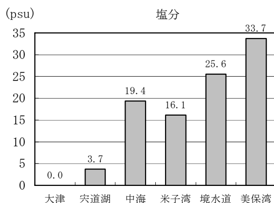
図 3.2-9 水域別の塩分(平成元～18年の全層平均)
