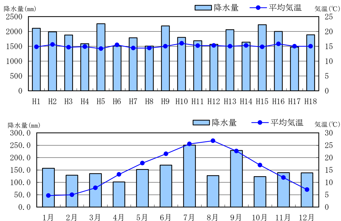
図 3.1-5 気温・降水量の変化(松江气象台、平成元～18年の平均)
