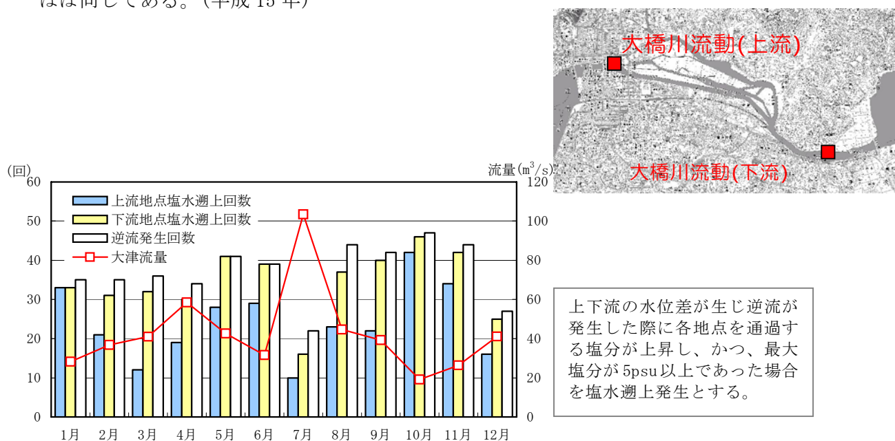
図 3.2-19 大橋川各地点の塩水遡上回数(平成 15 年)
