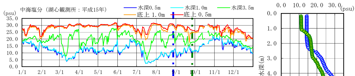
図 3.2-15 中海塩分の季節変化（平成 15 年）
