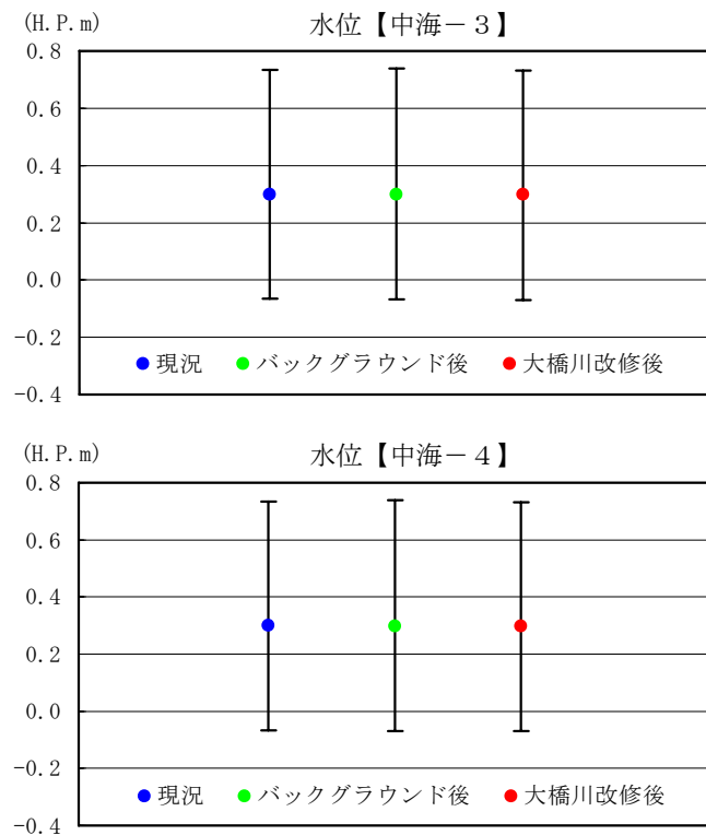
図 6.1.3-19 現況及び大橋川改修後の水位(10ヶ年平均・最大・最小)
