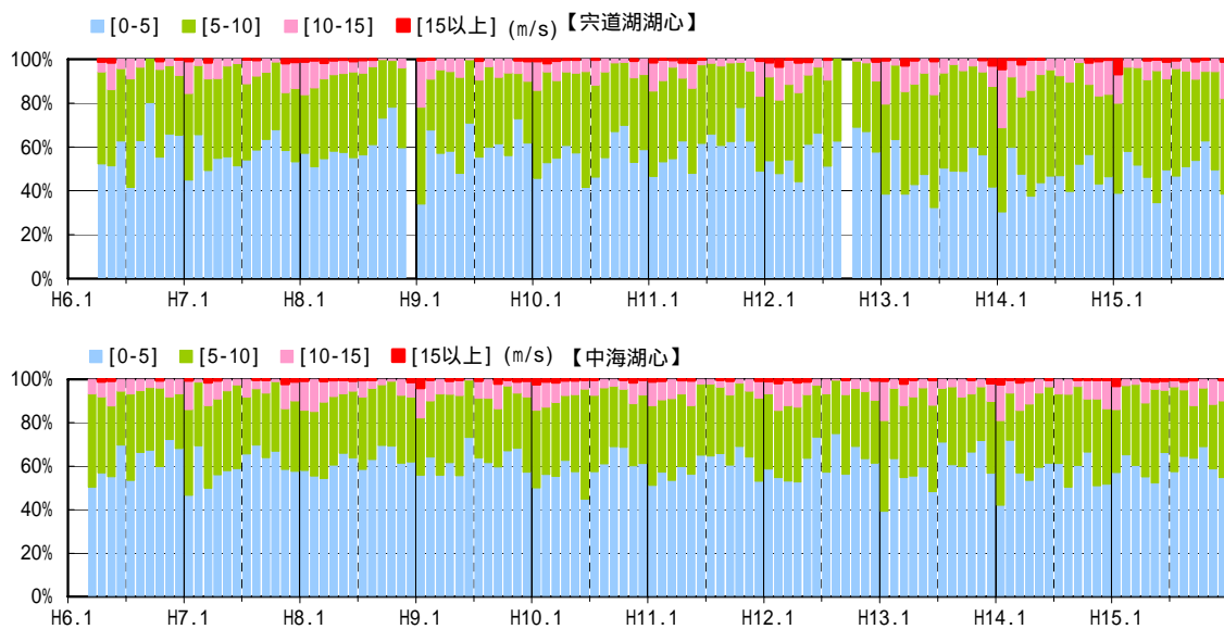
図 3.1-7 月別の風速頻度分布(平成 6 年～15 年)
