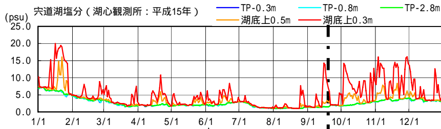
図 3.2-12 宍道湖塩分の季節変化 (平成 15 年)
