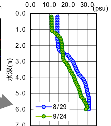
図 3.2-16 塩分鉛直分布
