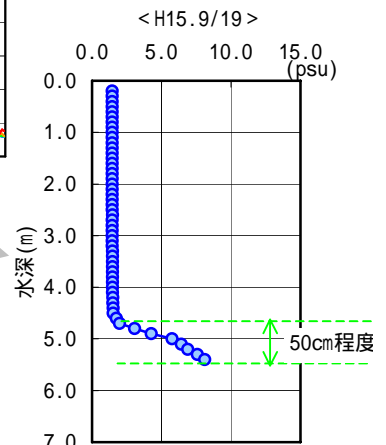
図 3.2-13 塩分鉛直分布
