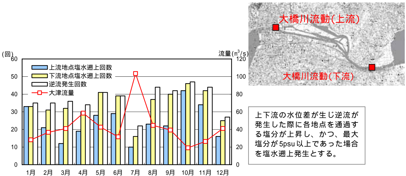
図 3.2-19 大橋川各地点の塩水遡上回数(平成 15 年)
