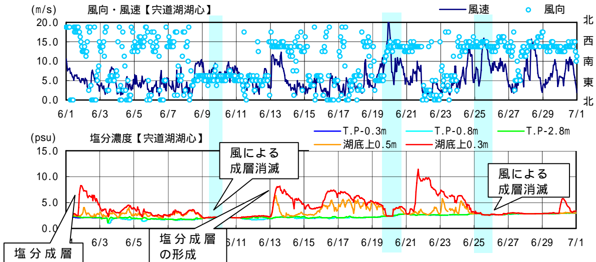
図 3.2-14 宍道湖塩分成層の風による消滅 (平成 15 年 6 月)
