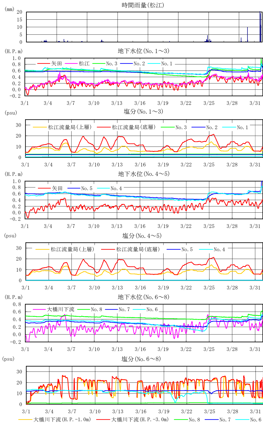
図 6. 1. 3-7 地下水調査結果【大橋川周辺，高潮時(H19. 3)】
