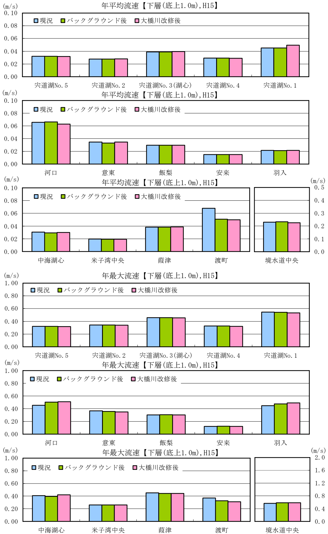
図 6. 1. 2-12 現況及び大橋川改修後の湖内流速【H15】
