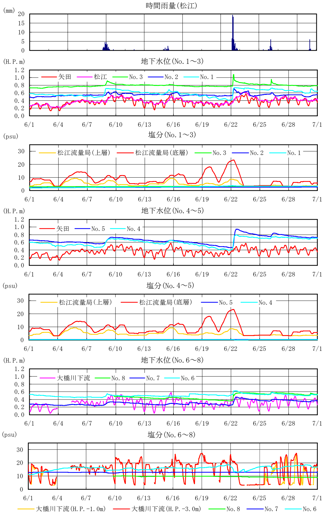
図 6. 1. 3-5 地下水調査結果【大橋川周辺，洪水時(H18. 6)】
