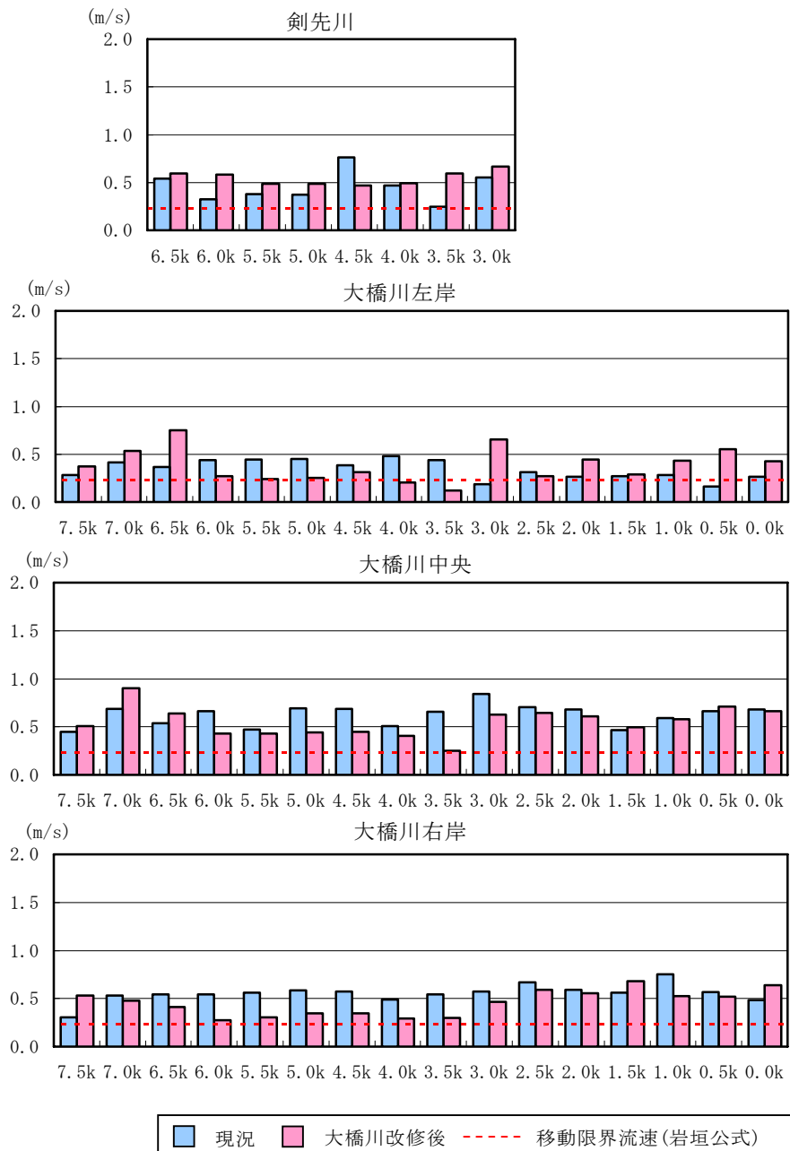
図 6.1.2-9 現況及び大橋川改修後の大橋川内流速【平常時(H6.7-9)】
