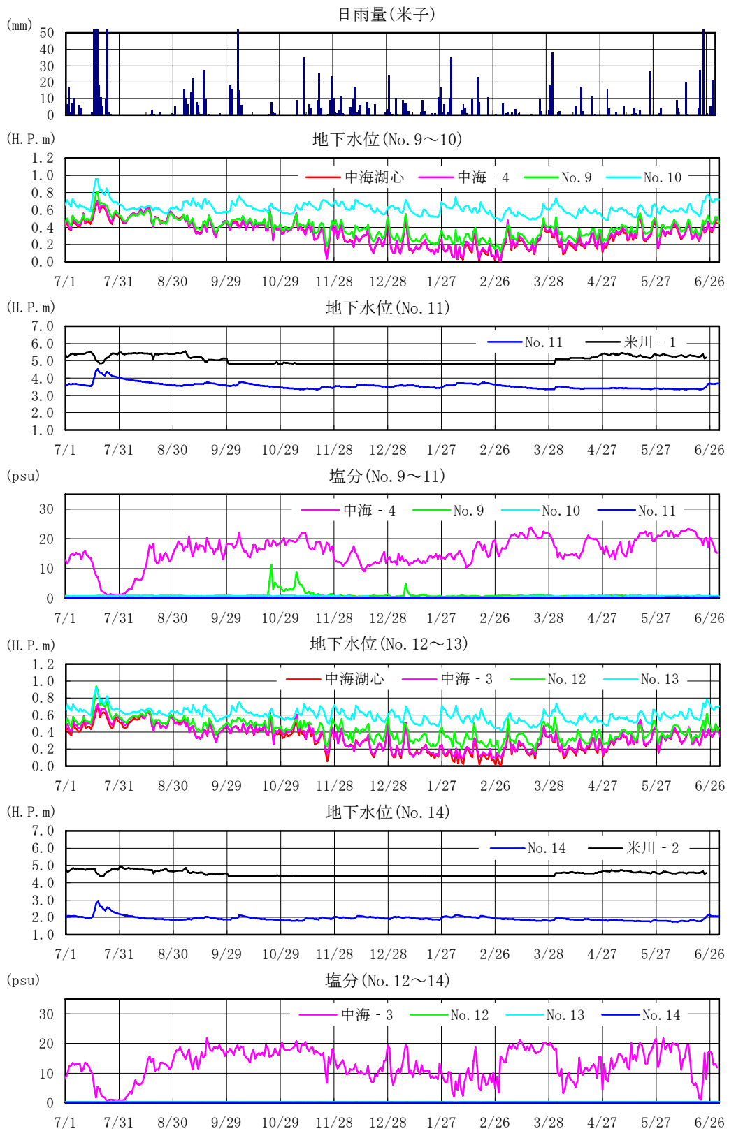
図 6.1.3-4 地下水調査結果
