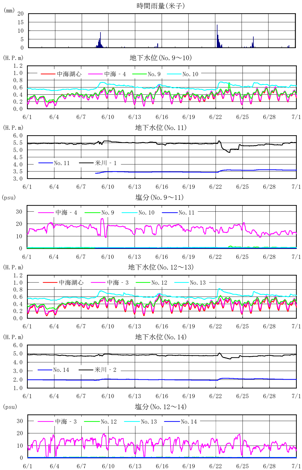
図 6. 1. 3-6 地下水調査結果【境港市～米子市（弓浜半島）地域，洪水時(H18. 6)】
