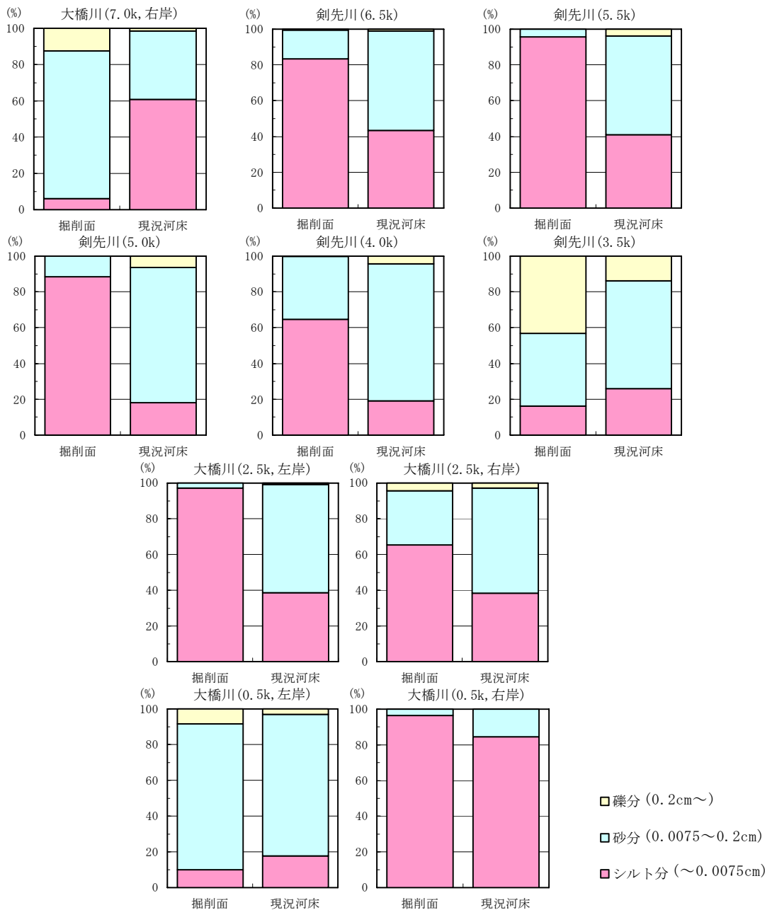
図 6.1.2-3 大橋川現況河床及び改修後掘削面の底質の粒径別質量割合
