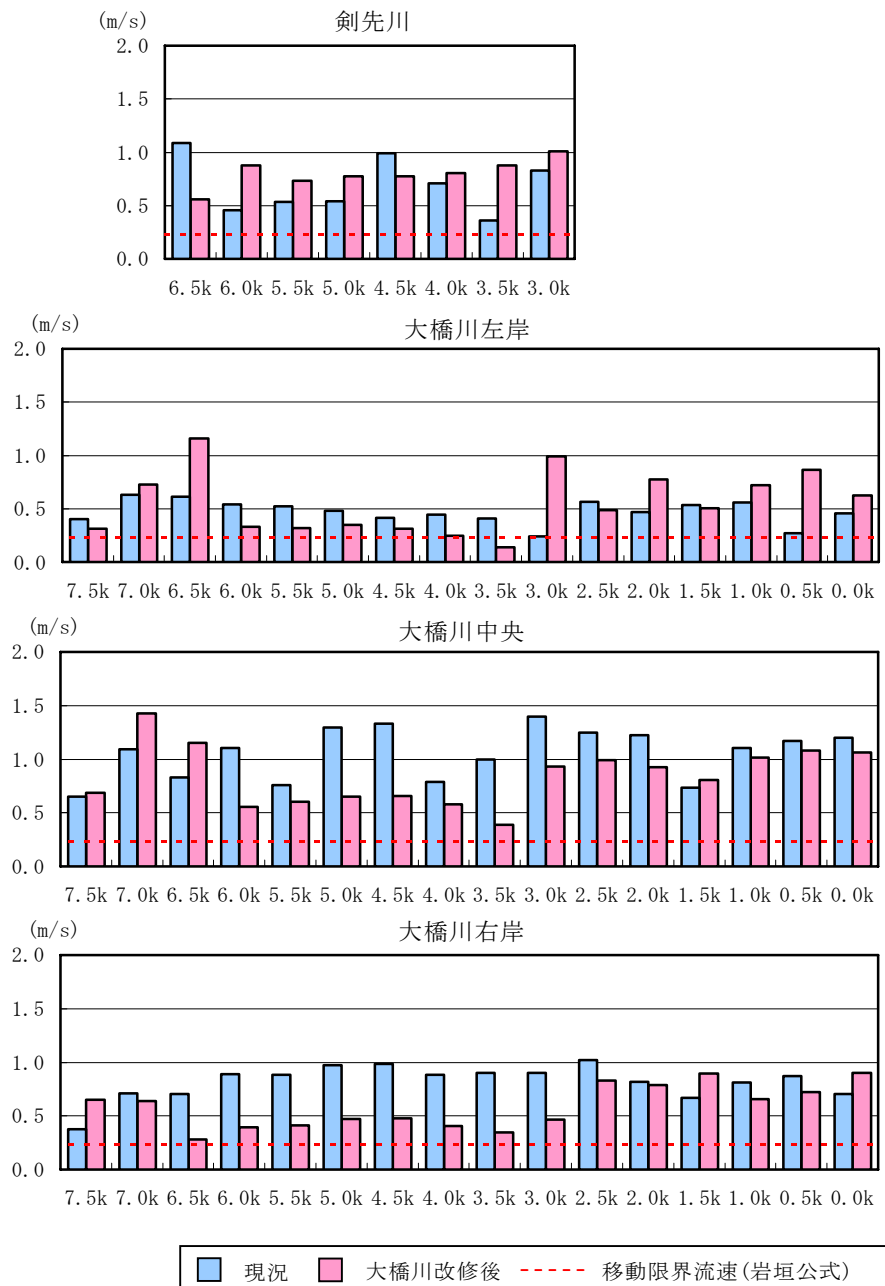
図 6. 1. 2-7 現況及び大橋川改修後の大橋川内流速【洪水時 (H9. 7)】
