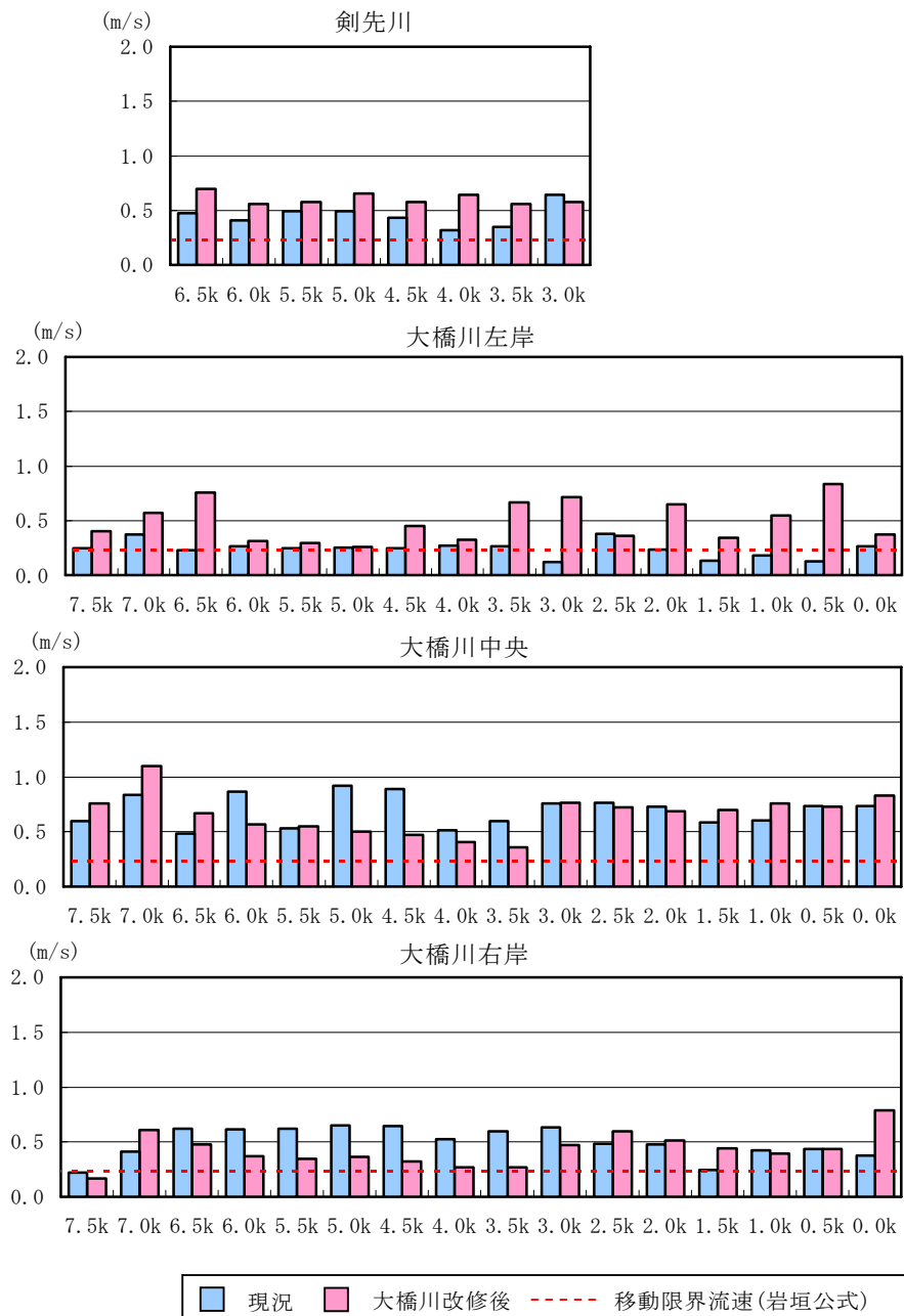
図 6. 1. 2-8 現況及び大橋川改修後の大橋川内流速【高潮時 (H14. 9)】
