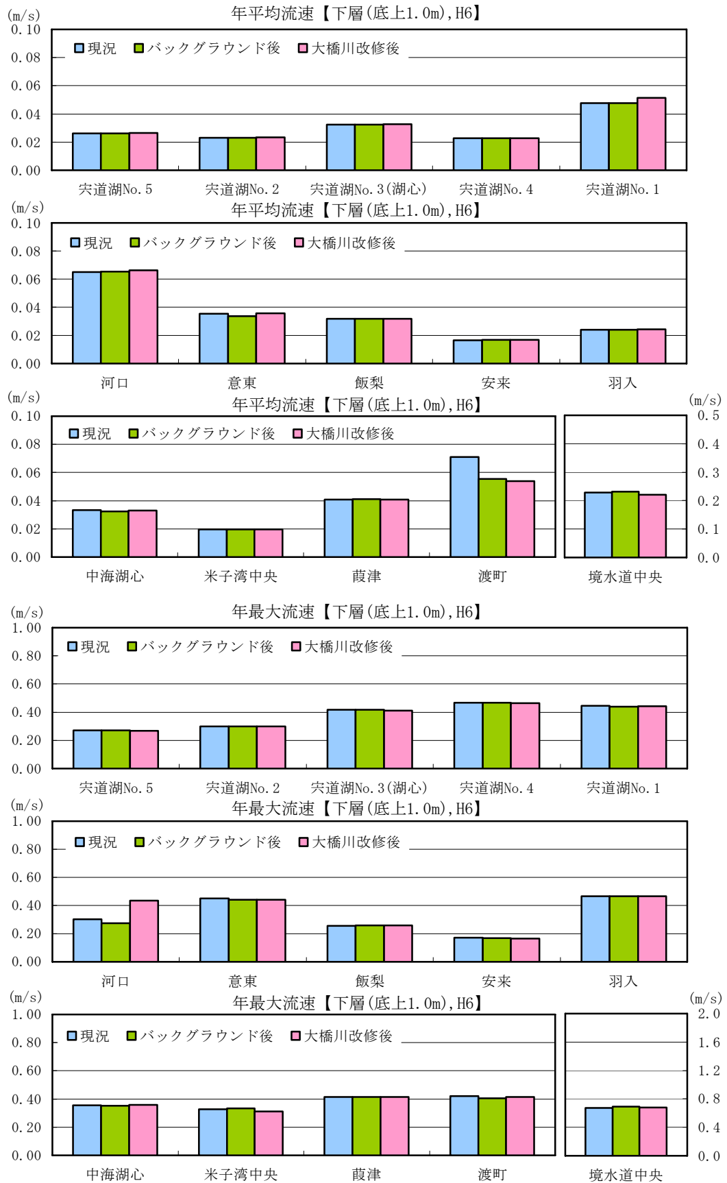
図 6. 1. 2-10 現況及び大橋川改修後の湖内流速【H6】
