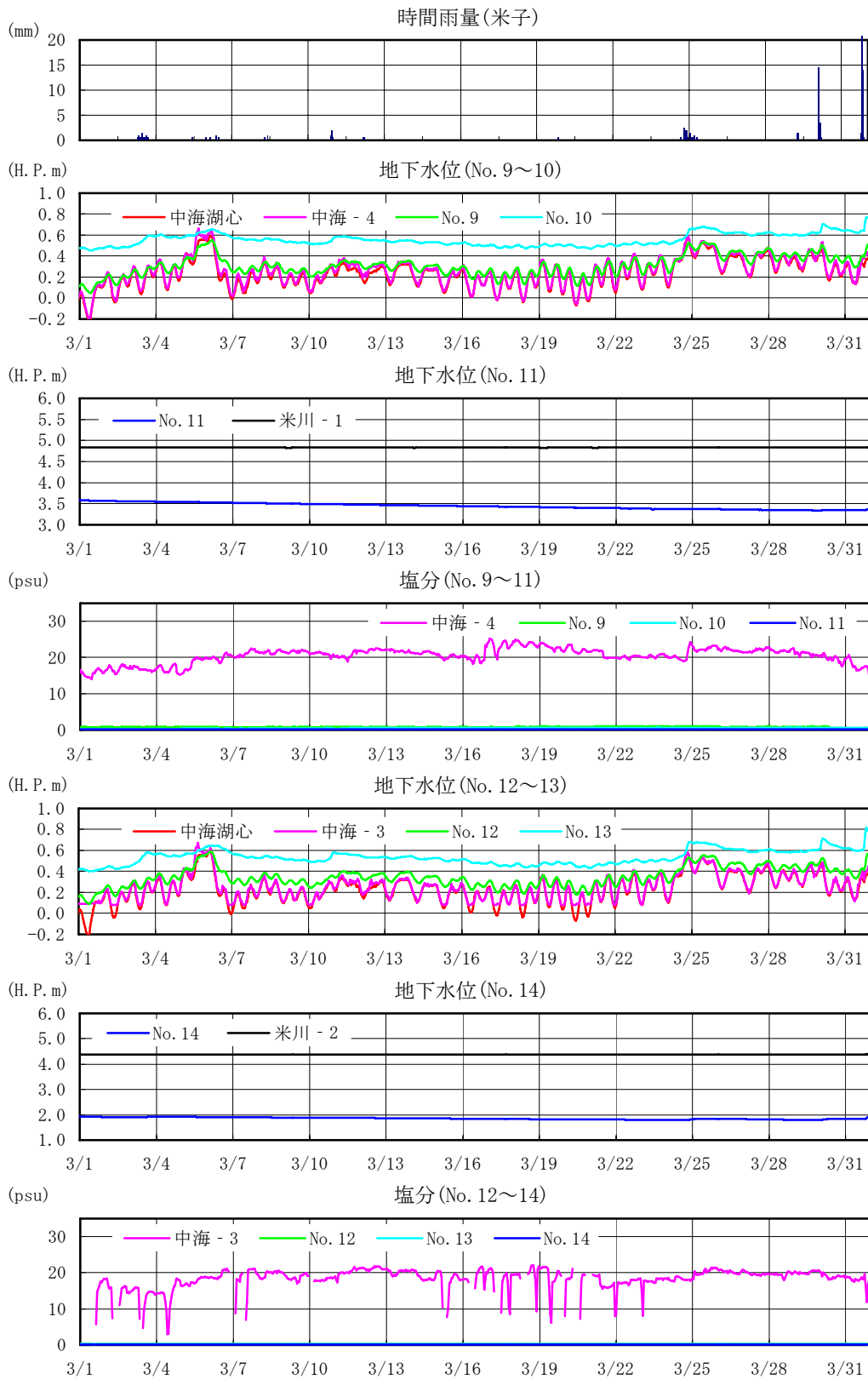
図 6.1.3-8 地下水調査結果【境港市～米子市（弓浜半島）地域，高潮時(H19.3)】
