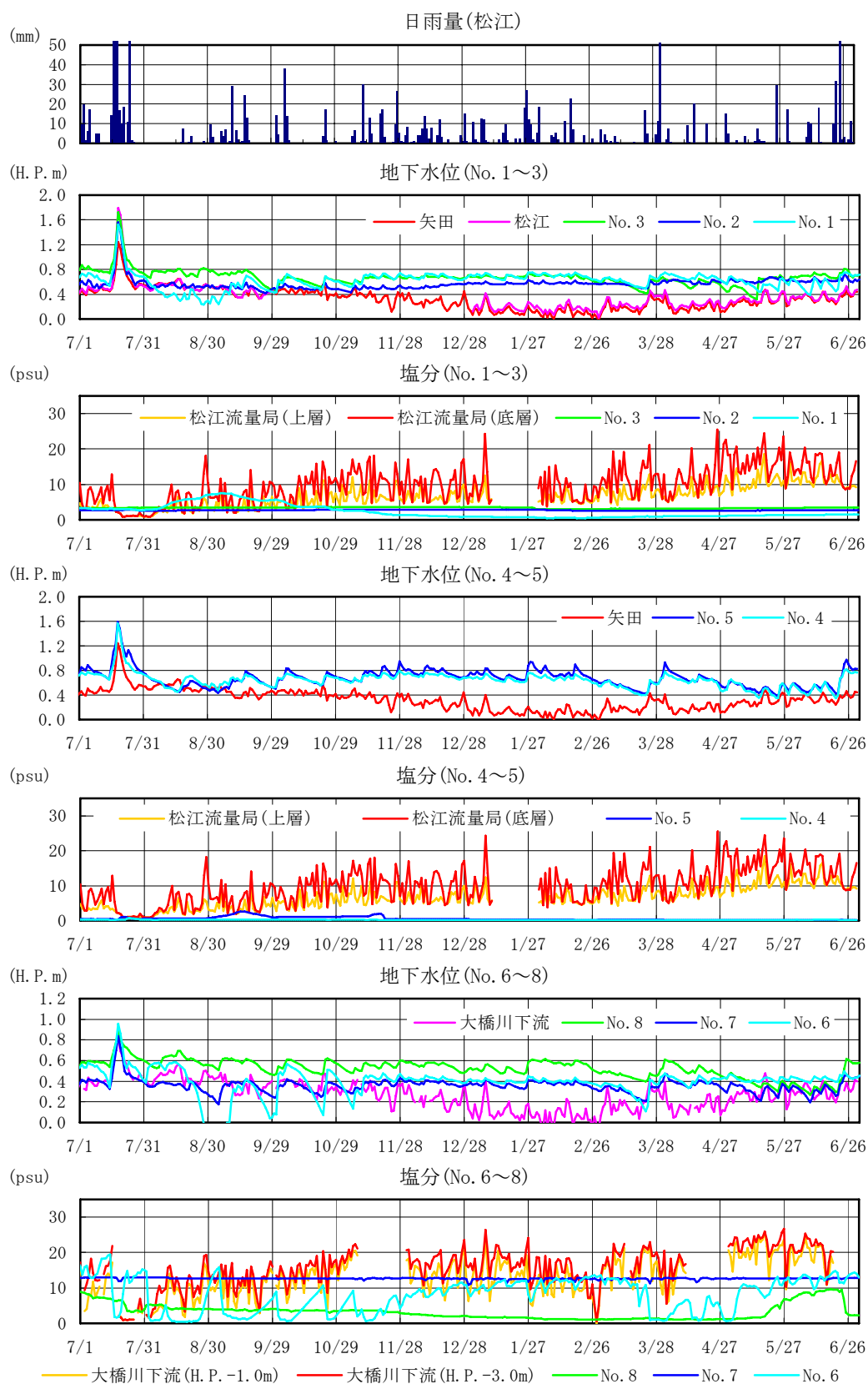
図 6.1.3-3 地下水調査結果【大橋川周辺, 日変動, H18.7/1~H19.6/30】
