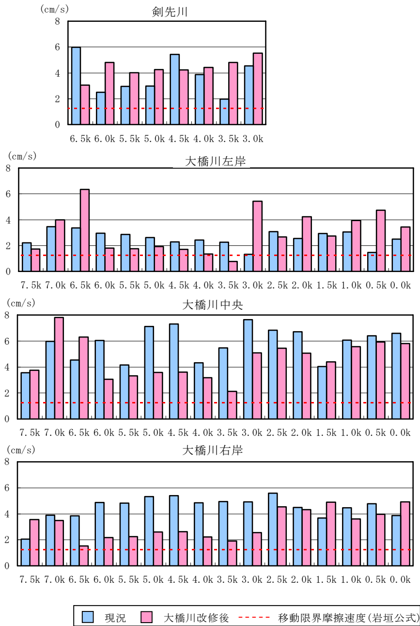
図 6. 1. 2-4 現況及び大橋川改修後の大橋川内摩擦速度【洪水時 (H9. 7)】
