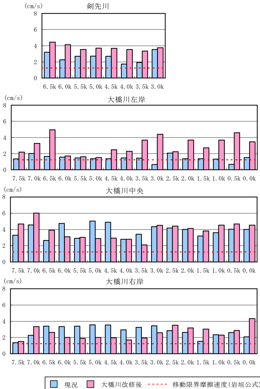
図 6.1.2-5 現況及び大橋川改修後の大橋川内摩擦速度【高潮時(H14.9)】
