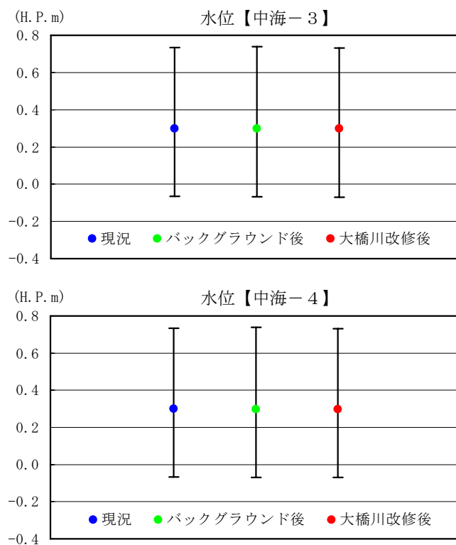
図 6.1.3-18 現況及び大橋川改修後の水位【10ヶ年平均】
