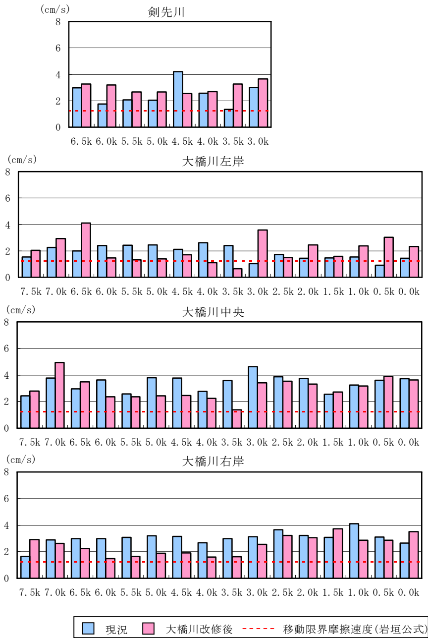
図 6.1.2-6 現況及び大橋川改修後の大橋川内摩擦速度【平常時(H6.7-9)】
