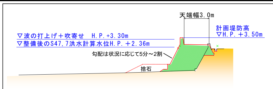
図 5-18 整備イメージ図（横断図）
