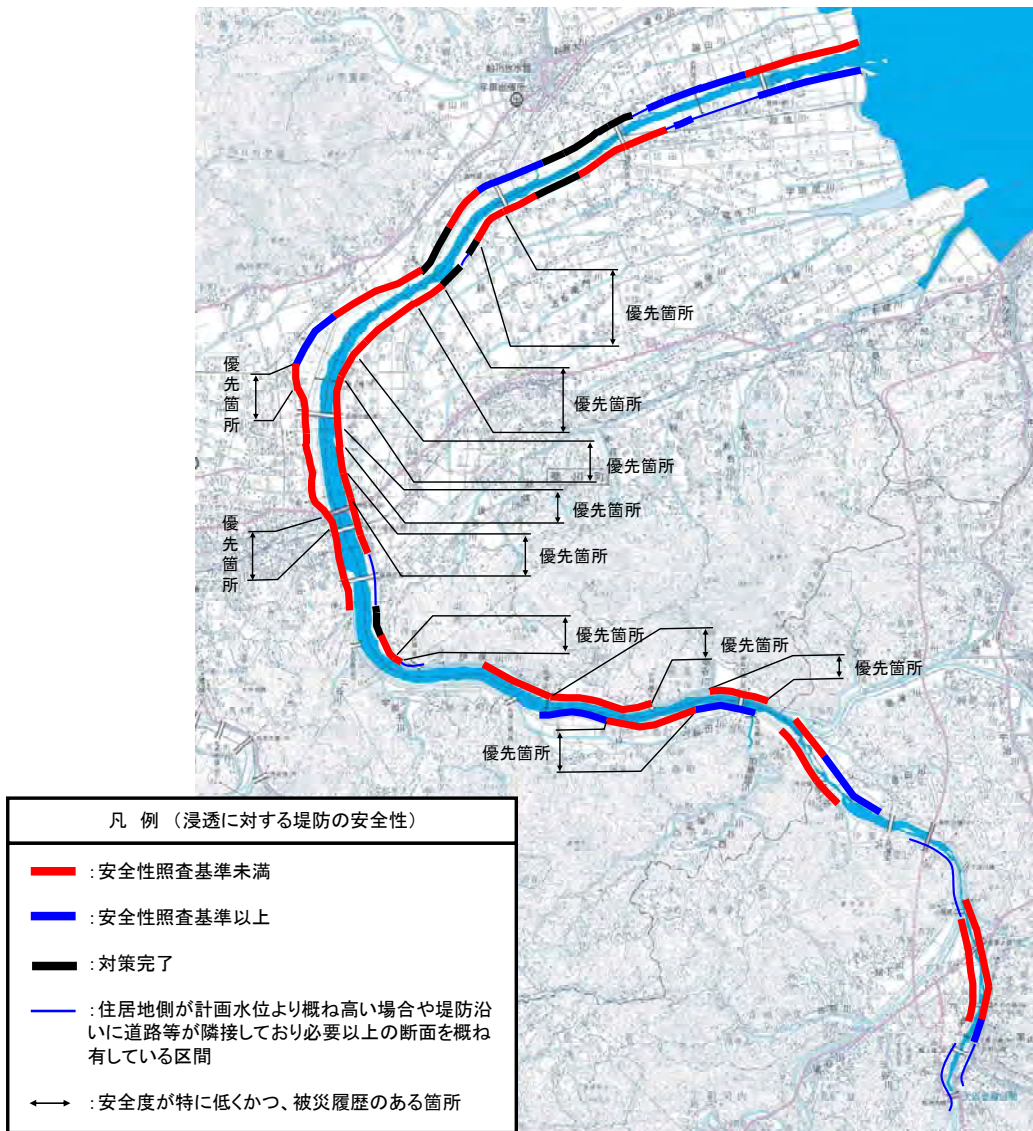
図 3-5 堤防詳細点検結果
