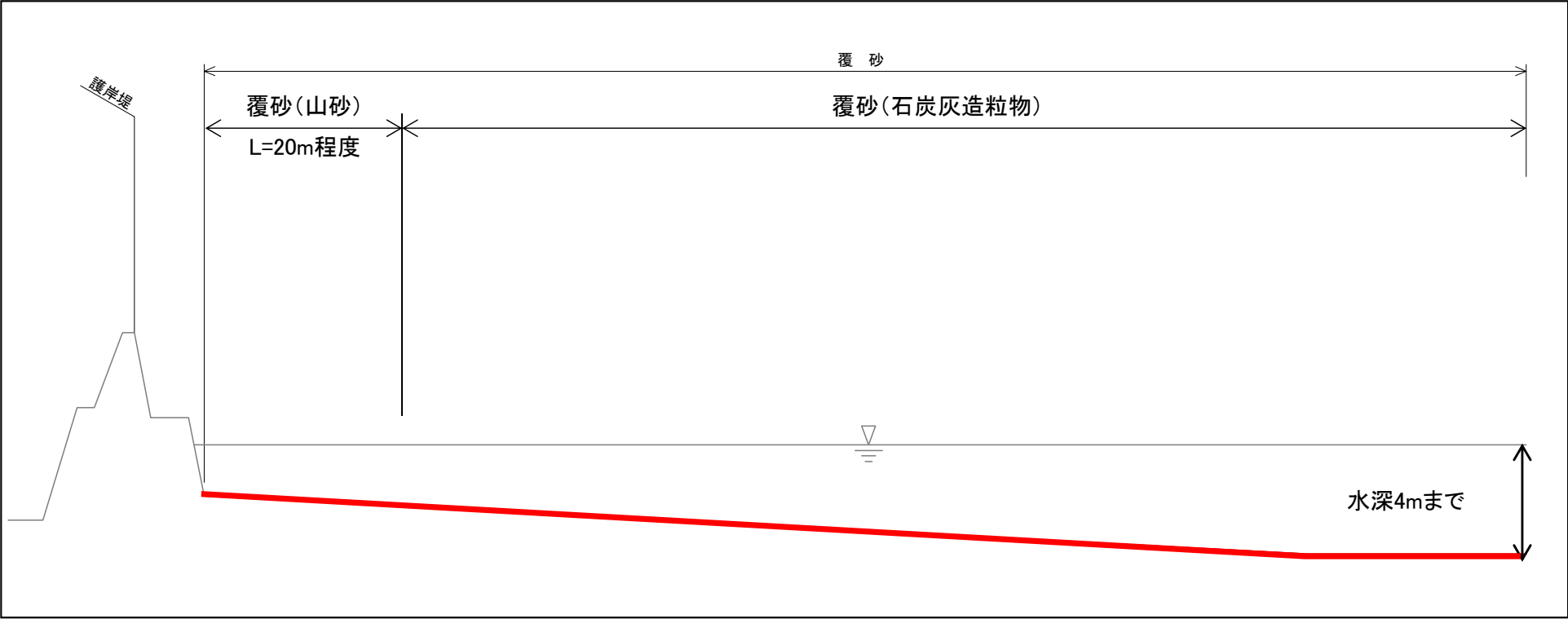
覆砂拡大図
