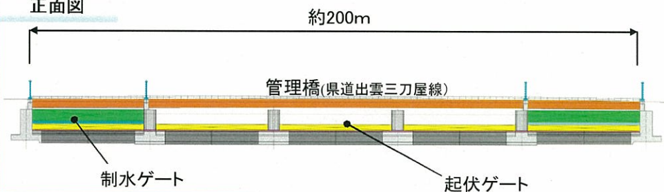
正面図
