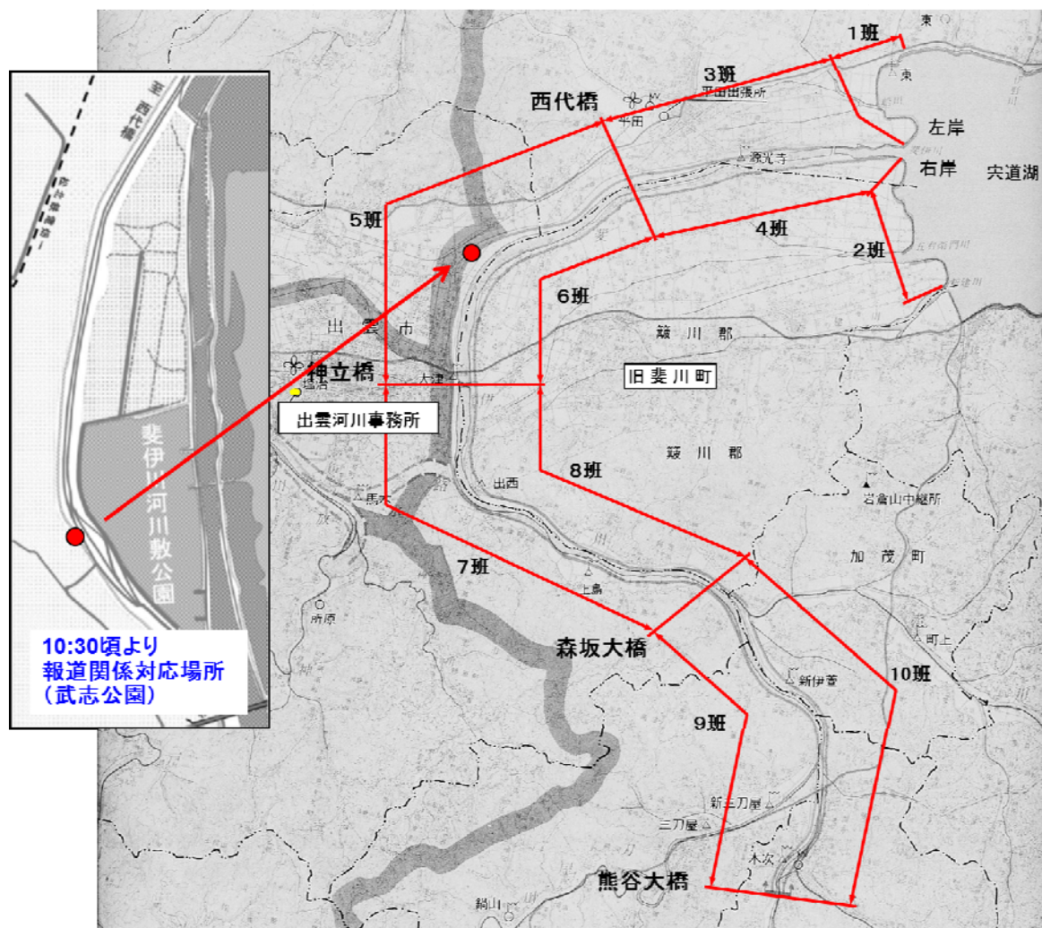
斐伊川河川堤防出水期前一斉堤防点検位置図
