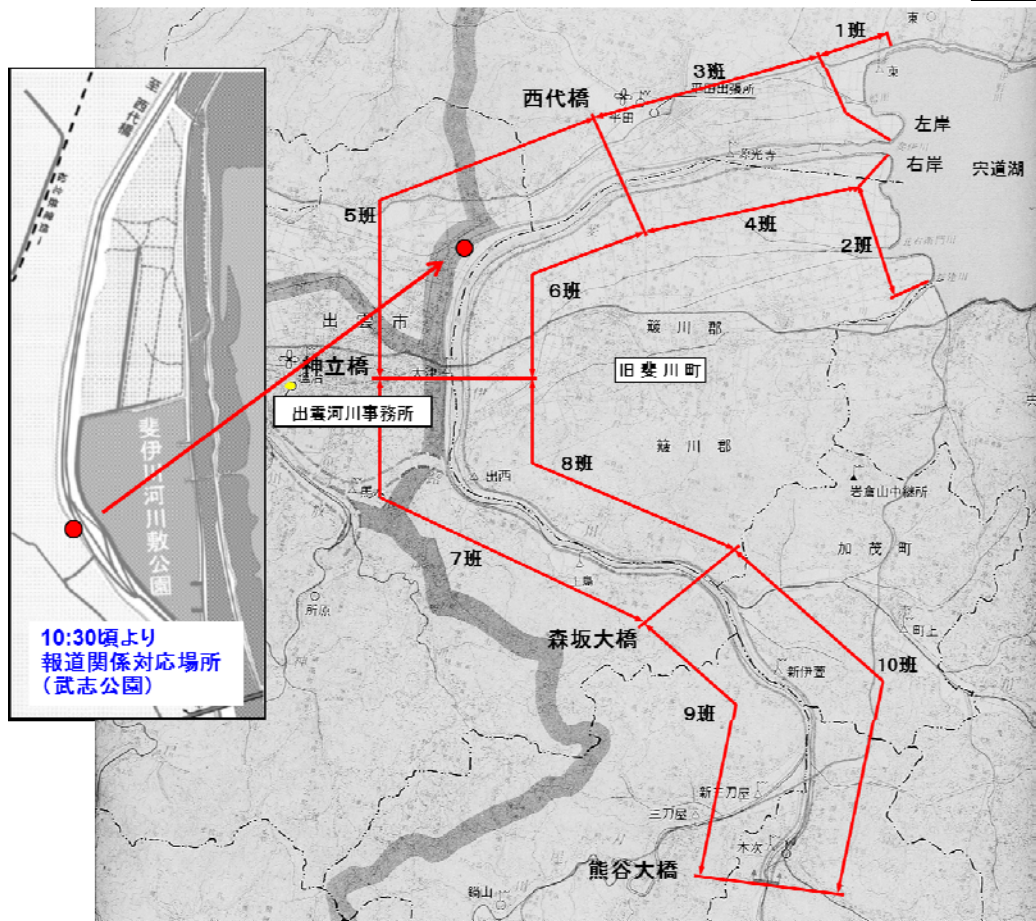
斐伊川河川堤防出水期前一齐堤防点検位置図
