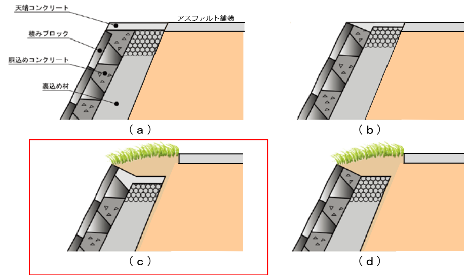
図1 天端処理(「出典:多自然川づくりポイントブックⅢ」に加筆)
