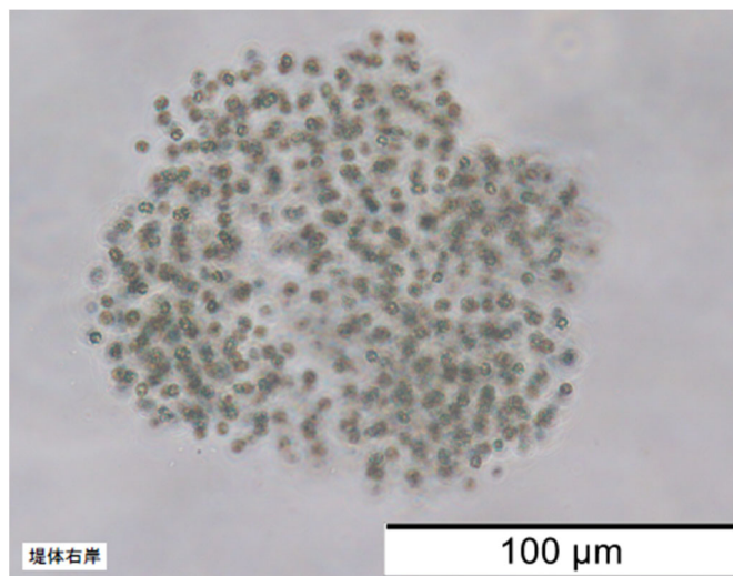
らんそう 藍藻類(ミクロキスティス) ※ 今回確認された顕微鏡写真
