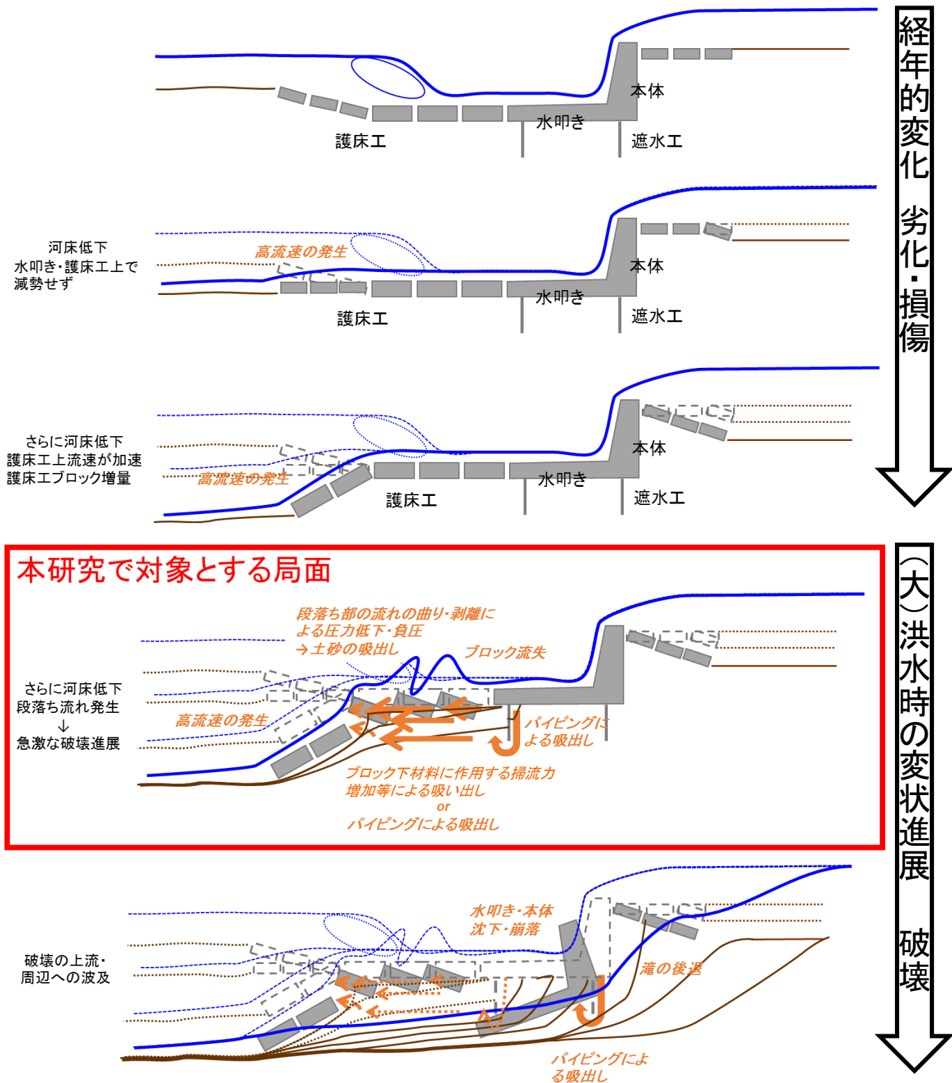
図-2 横断構造物の劣化・損傷・破壊のプロセス
