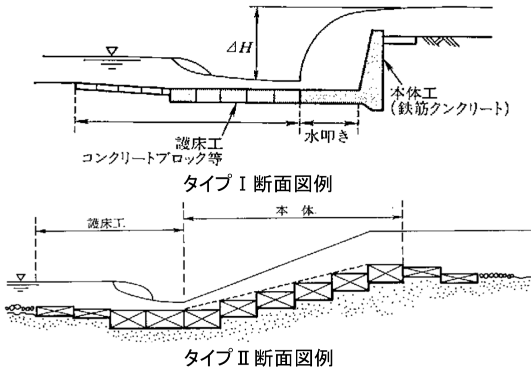
図－３ 横断構造物の構造タイプ（タイプⅠ、タイプⅡ）
