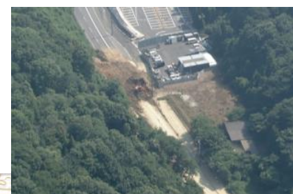
⑥ 尾道市美ノ郷町：土工用防護柵設置支援
