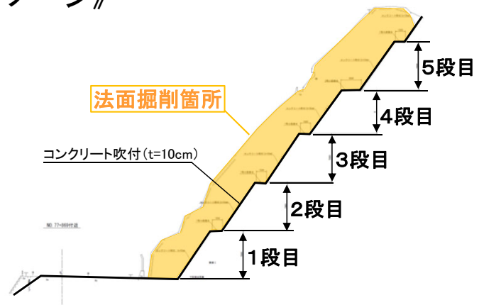
法面掘削
