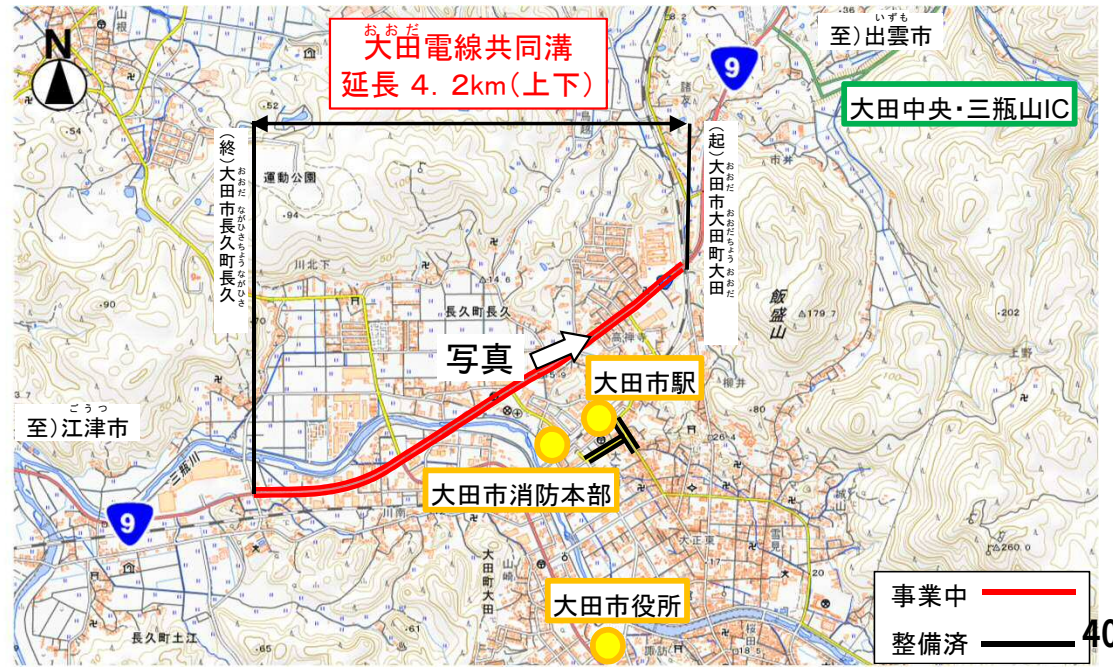
《平面図》
