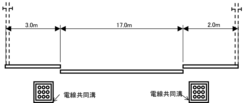
《標準横断図》
