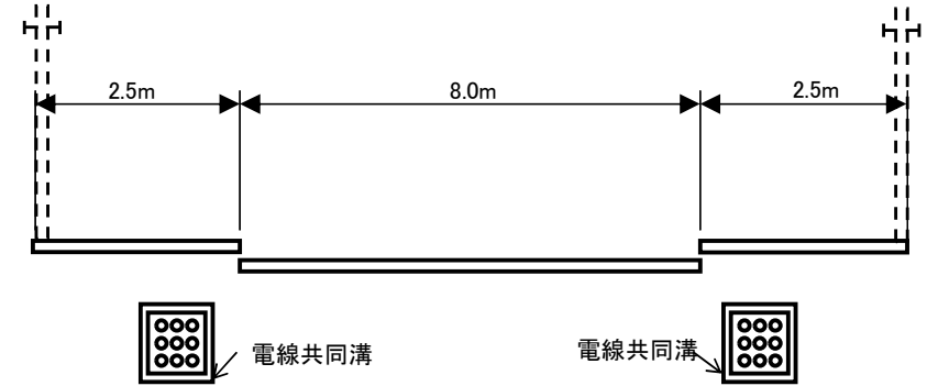
《標準横断図》
