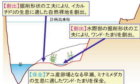
河川環境の保全・創出（河道掘削イメージ）
