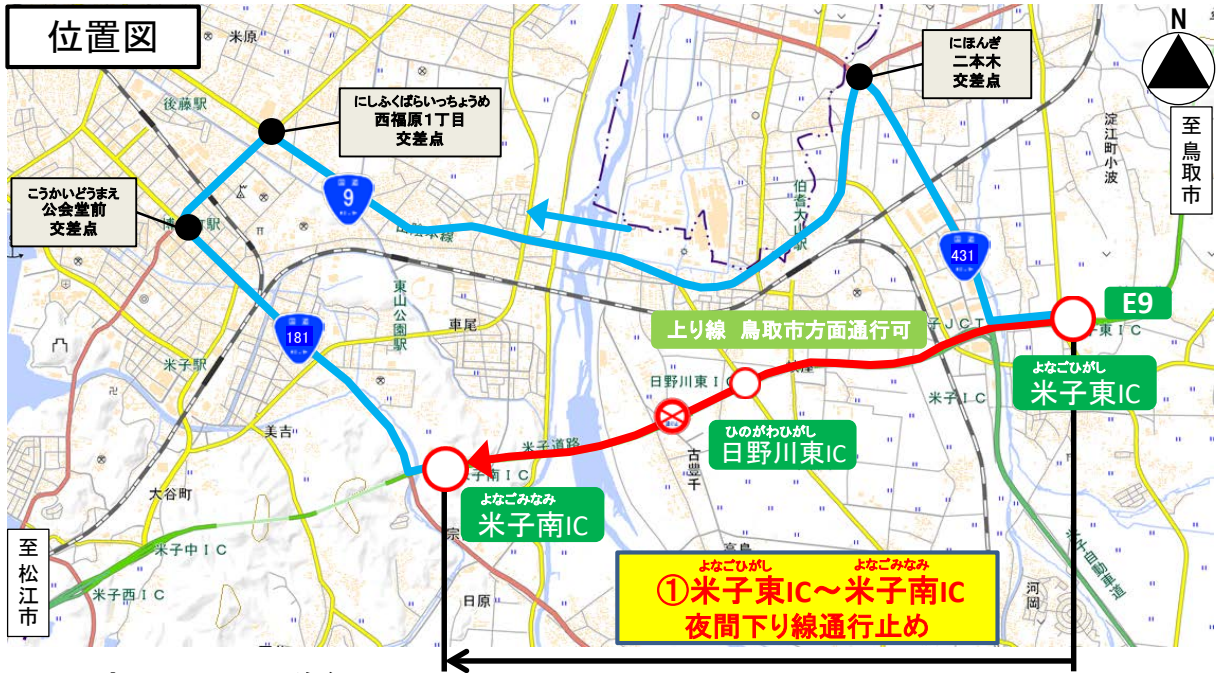
米子東IC周辺詳細図
