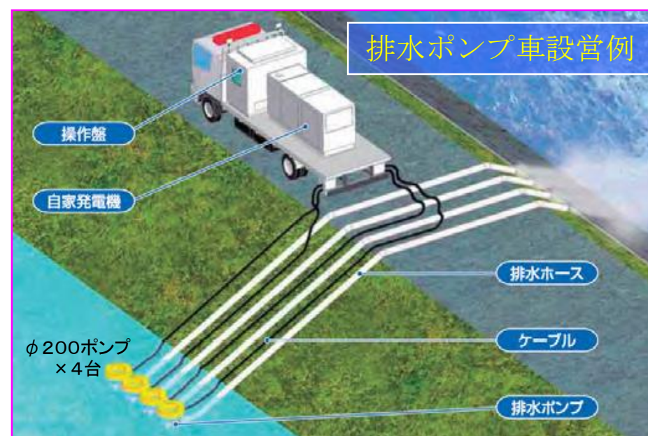
② 排水ポンプ車(30m 3 /min)
