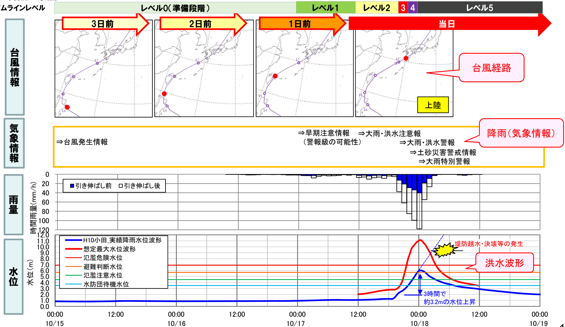
平成10年台風10号波形
