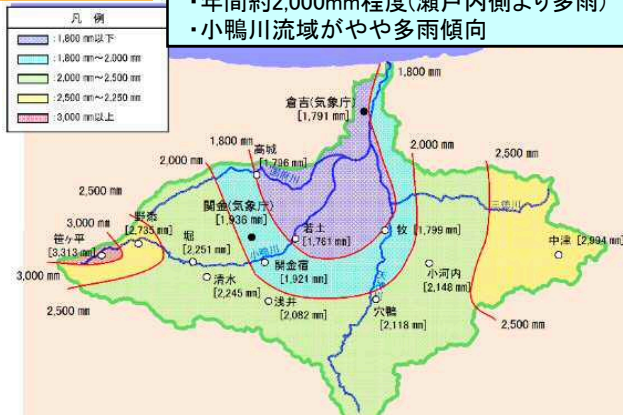
年間降雨量の分布(平成17年～平成30年)
