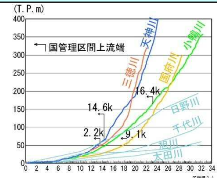
天神川と近傍河川の縦断面図
