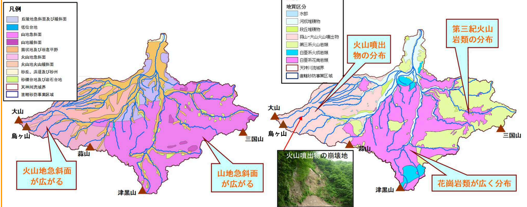
地質図（「20万分の1日本シームレス地質図データベース」 独立行政法人産業技術総合研究所 2005）
