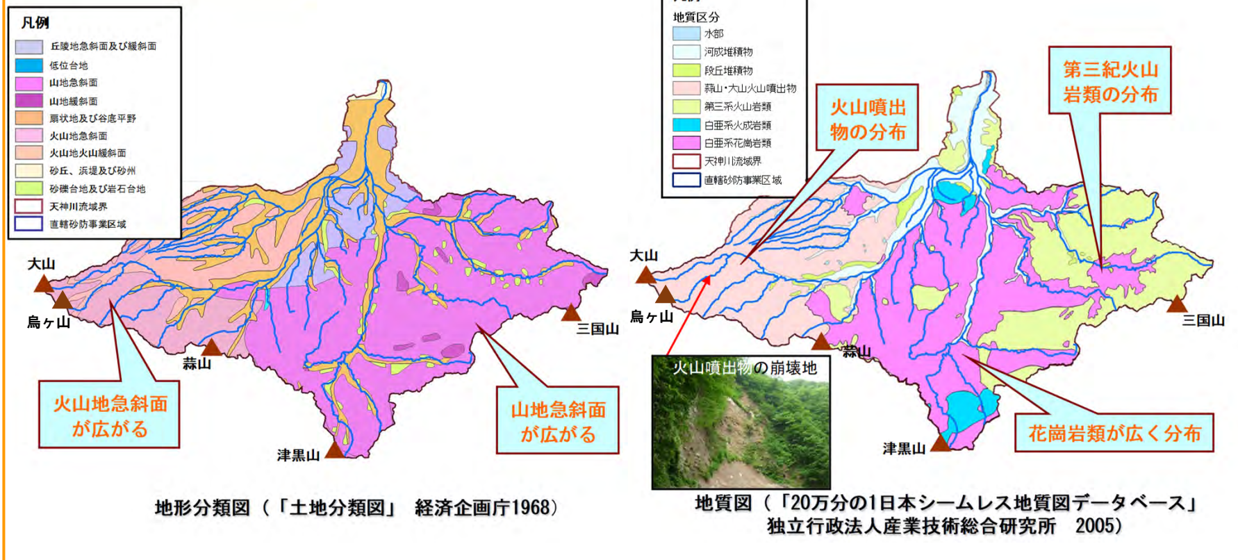
地形分類図および地質図
