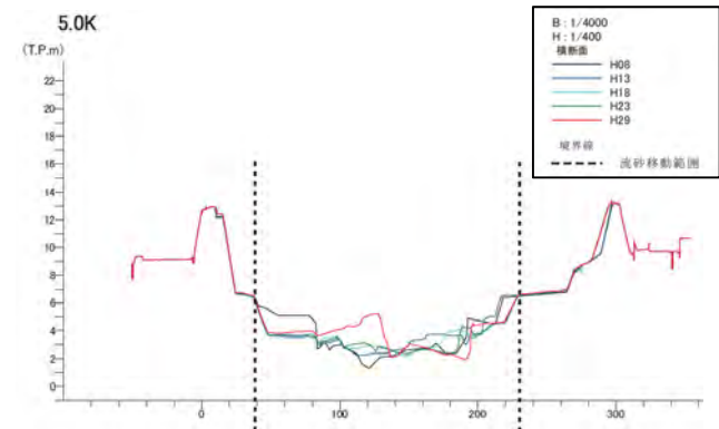
天神川5k000における平成8年以降の土砂堆積状況
