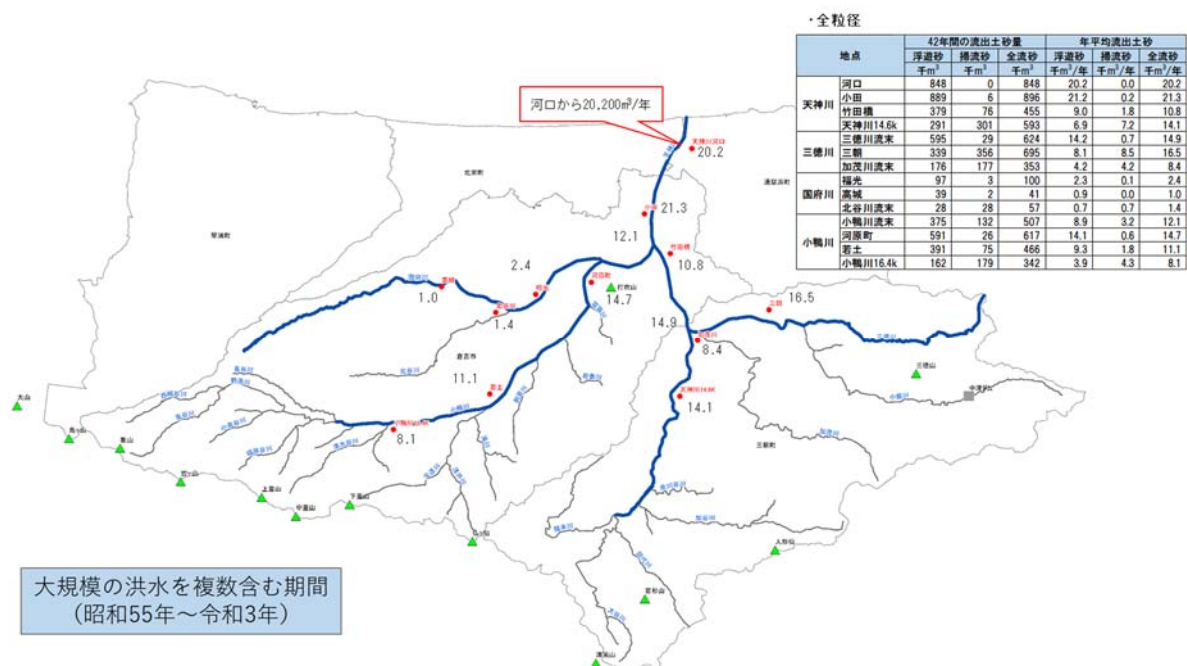
図 5.6-1 土砂動態マップ（全粒径）
