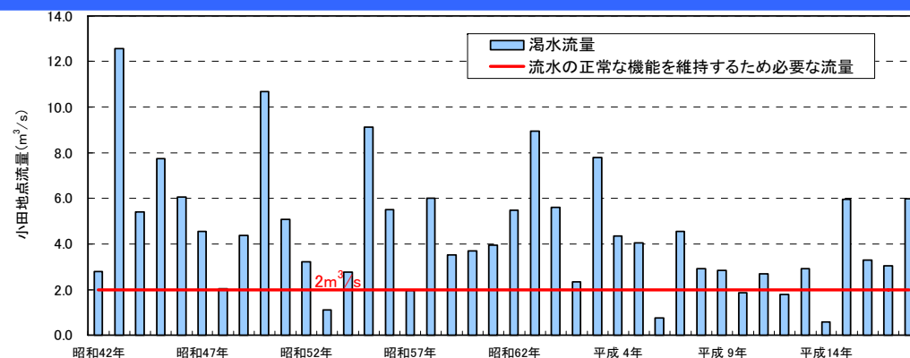
天神川小田地点における流況の経年変化
