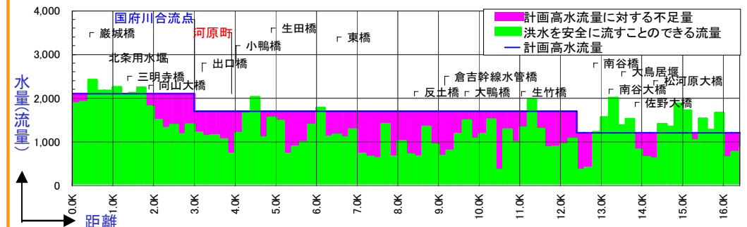
小鴨川流下能力図
