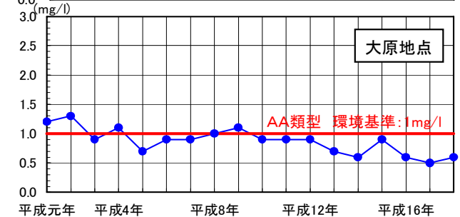
環境基準地点の水質(BOD75%値)経年変化
