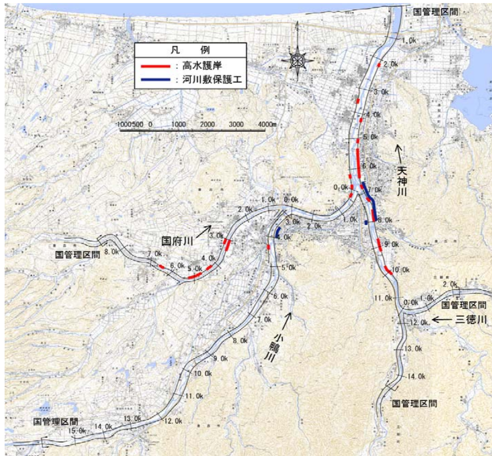
急流河川の侵食対策～高水護岸等の位置図～
