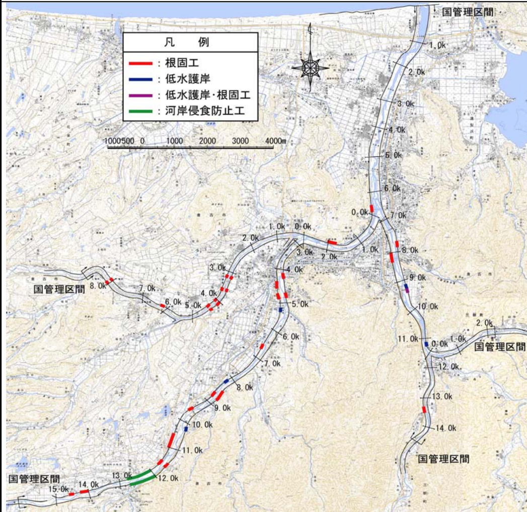
急流河川の侵食対策～根固工・低水護岸等を施工する箇所的位置図
