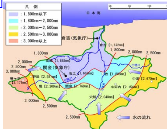
年間降水量の分布(平成6年～平成16年)
