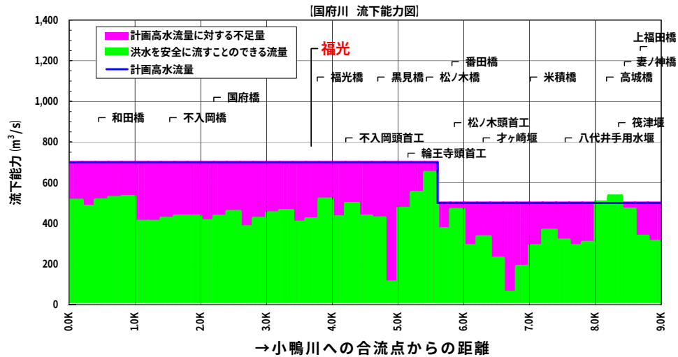
図 2.1.6 現在国府川が安全に流すことの出来る流量
