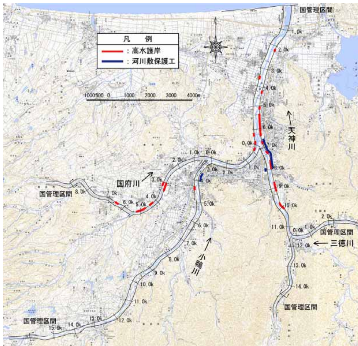
図 5.1.7 堤防侵食防止のため高水護岸等を施工する区間位置図
