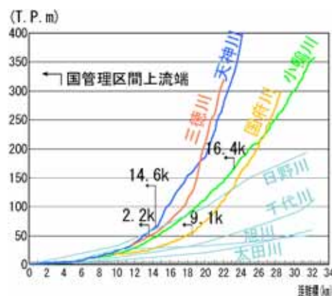
図5.1.7 天神川水系河川の河床勾配
