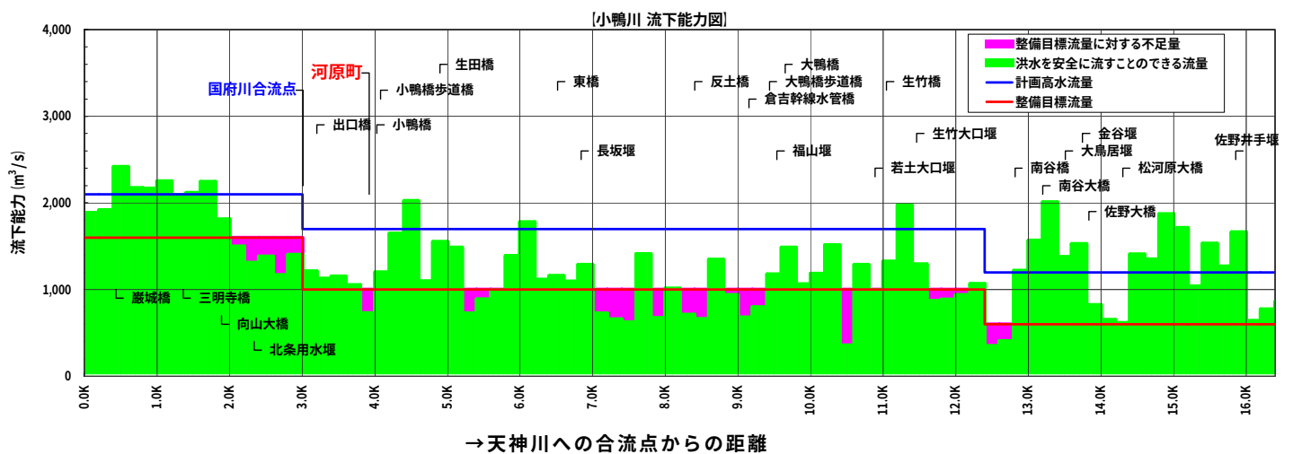
図 5.1.2 現在小鴨川が安全に流すことの出来る流量
