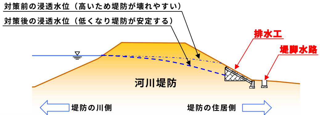
堤防強化対策工のイメージ図
