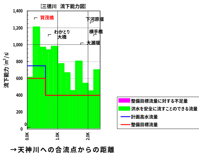
図 5.1.4 現在三徳川が安全に流すことの出来る流量
