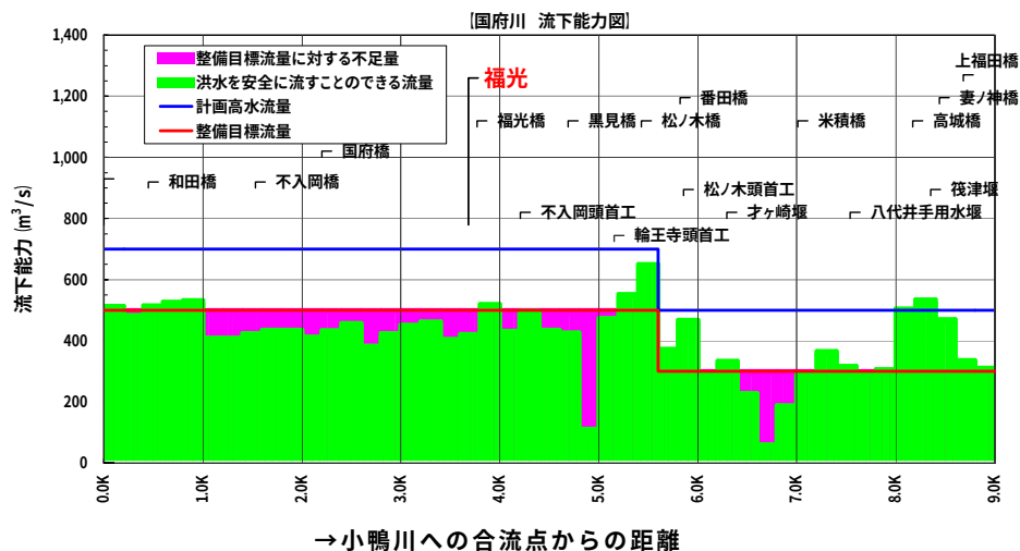
図 5.1.3 現在国府川が安全に流すことの出来る流量
