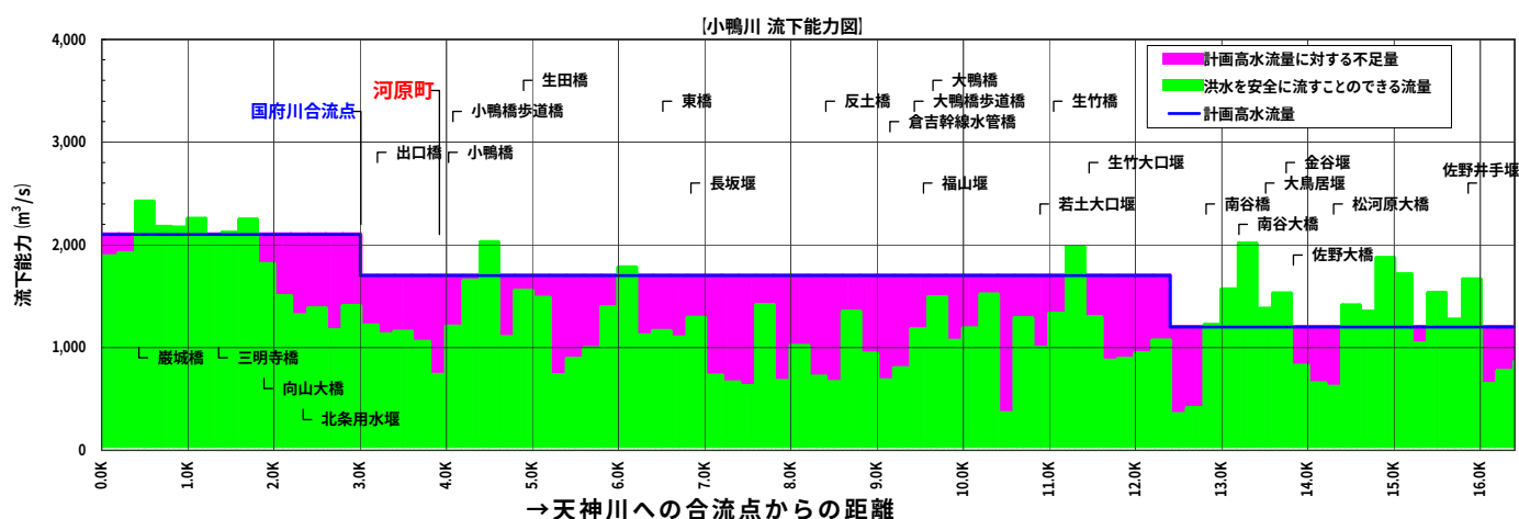
図 2.1.5 現在小鴨川が安全に流すことの出来る流量
