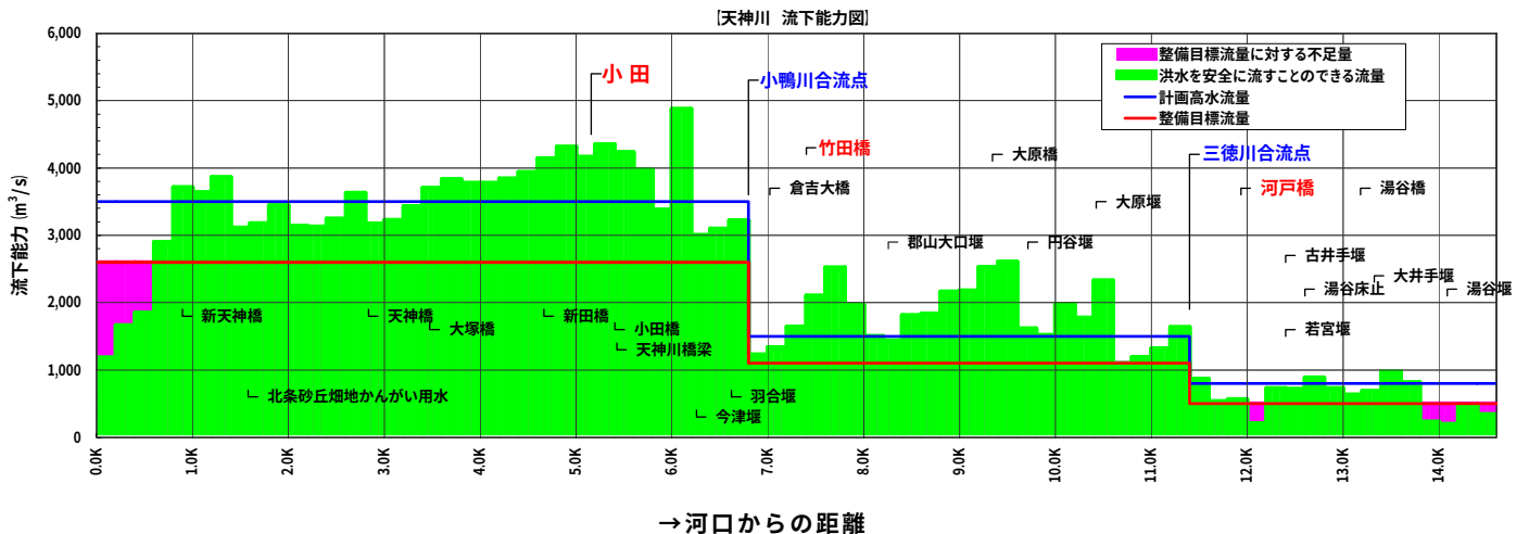
図 5.1.1 現在天神川が安全に流すことの出来る流量
