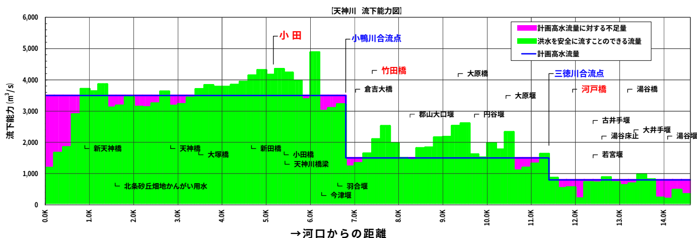
図 2.1.4 現在天神川が安全に流すことの出来る流量
