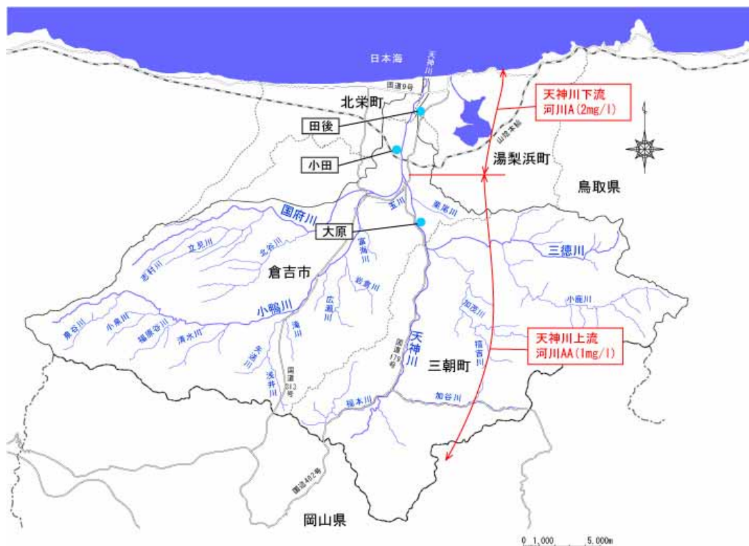
図 2.2.3 水質環境基準点及び類型指定区間
