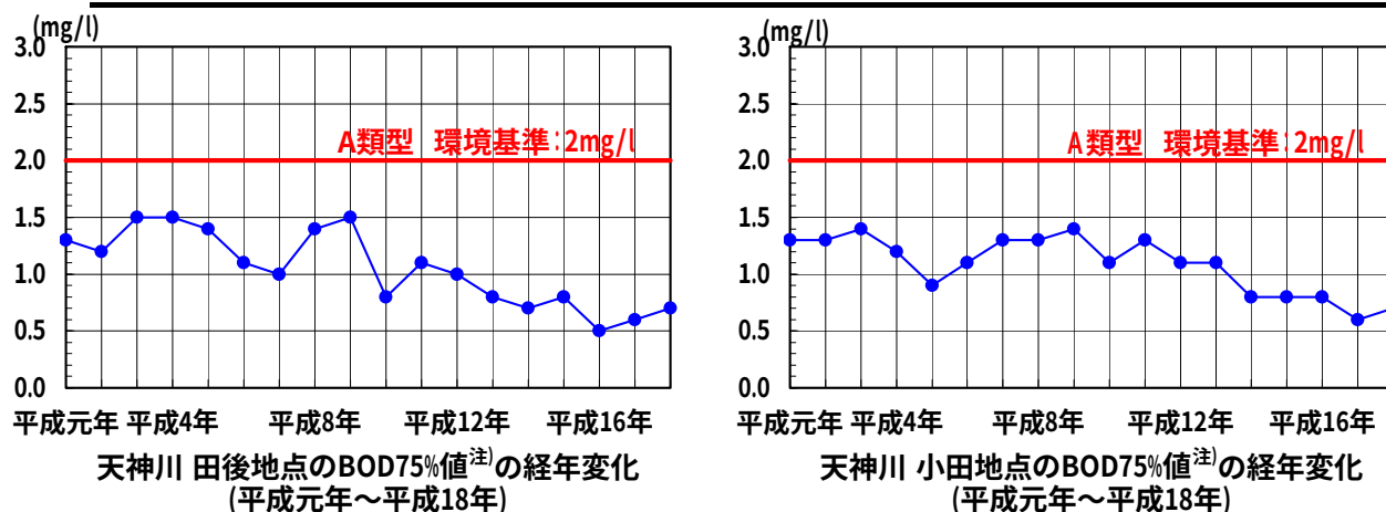
図 2.2.4 天神川：田後地点及び小田地点における水質の経年変化
