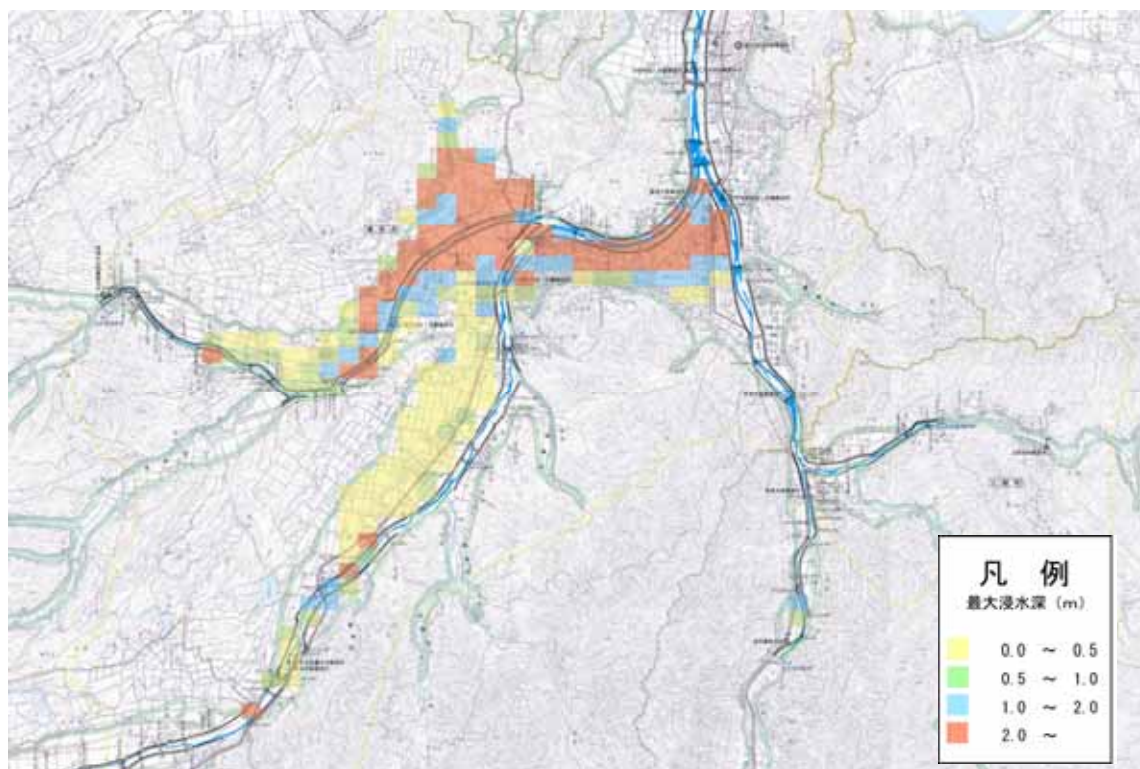
図 1.2.1 昭和 34 年伊勢湾台風洪水による浸水想定区域 注 1)
