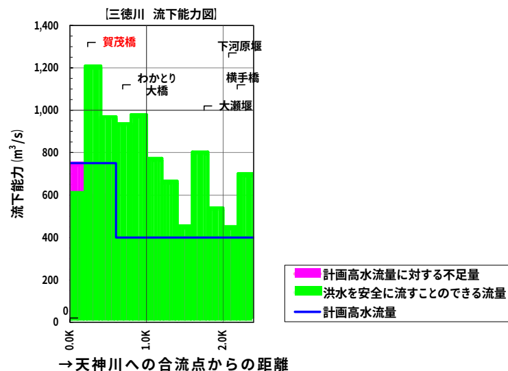
図 2.1.7 現在三徳川が安全に流すことの出来る流量
