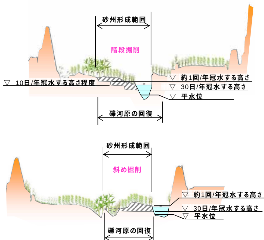
図 5.1.9 礫河原再生のための河床掘削イメージ (イメージであり実際の掘削形状は異なることがあります)
