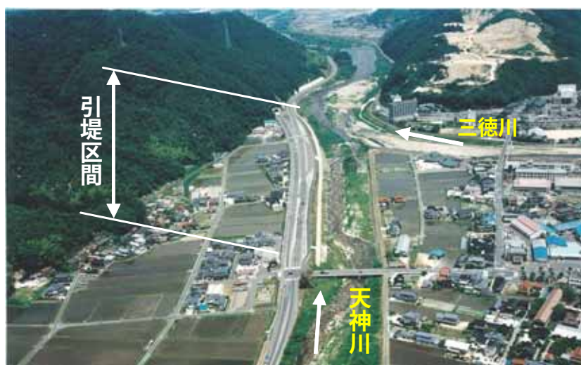
近年の治水事業の例：完成した若宮箇所改修事業（平成 17 年撮影）
