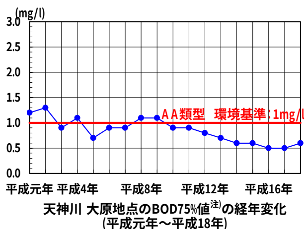
図 2.2.5 天神川：大原地点における水質の経年変化
