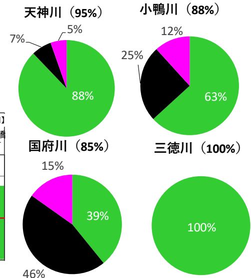
各河川の流下能力達成率
