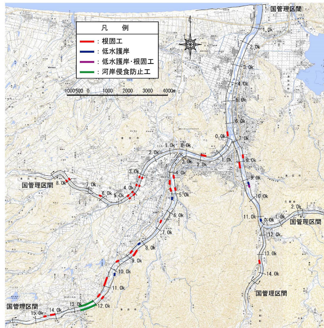
図 5.1.8 河岸侵食防止のため低水護岸・根固工・河岸侵食防止対策工を施工する区間位置図
