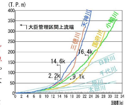
図 2.1.1 天神川水系河川の河床勾配
