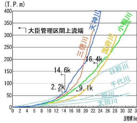
図 5.1.2 天神川水系河川の河床勾配
