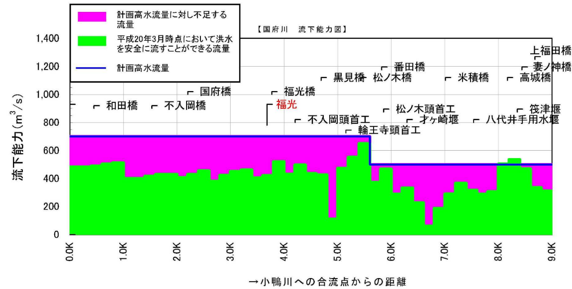
図 2.1.6 現在国府川が安全に流すことの出来る流量
