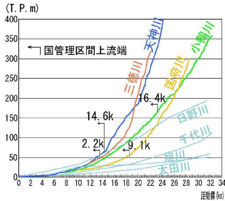
図 5.1.7 天神川水系河川の河床勾配
