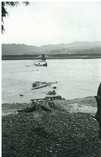
昭和 34 年伊勢湾台風洪水 大塚橋の流失状況
