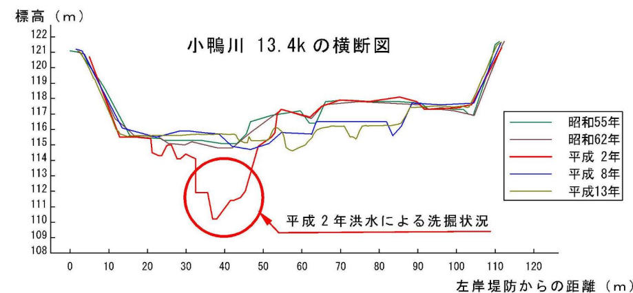
図 2.1.3 平成 2 年洪水における小鴨川の河床洗掘状況
