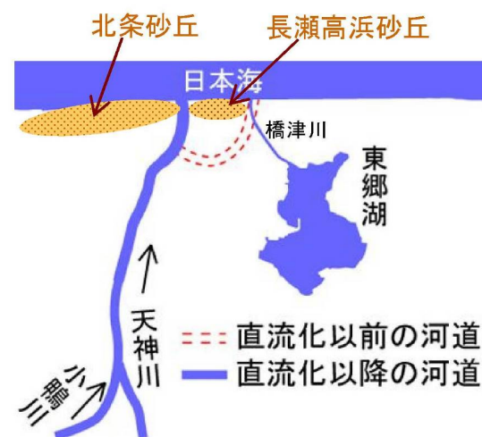
図 1.2.2 元文年間頃の天神川の直流水工
