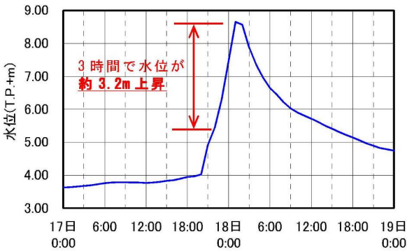
図 2.1.9 平成 10 年 10 月洪水による 水位の時間変化(小田)
