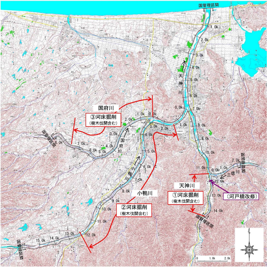
図 5.1.6 河積確保のための河道整備区間位置図
