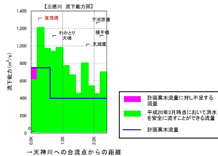
図 2.1.7 現在三徳川が安全に流すことの出来る流量
