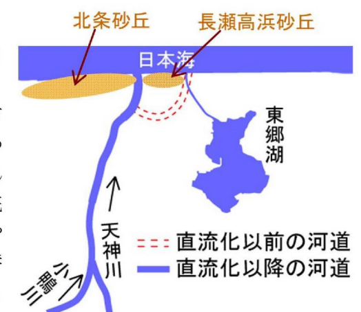
図 1.3.1 元文年間頃の天神川の直流水工
