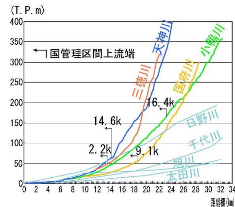
図 2.1.1 天神川水系河川の河床勾配
