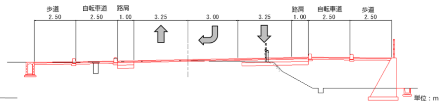
【計画断面図】
