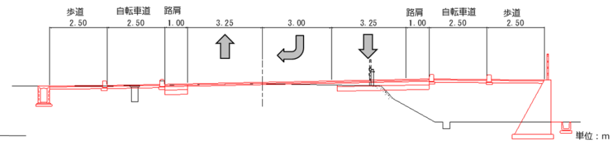
【計画断面図】
