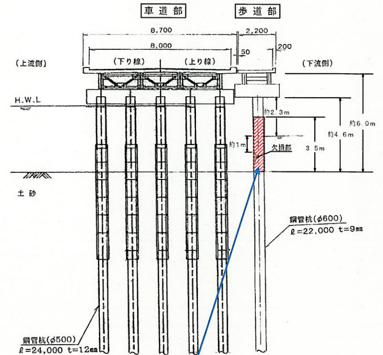
断面図
