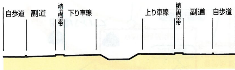
現況断面
