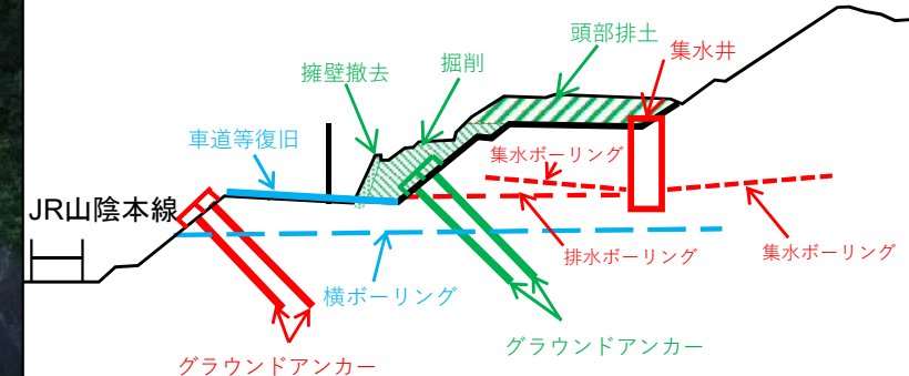
A-A断面
