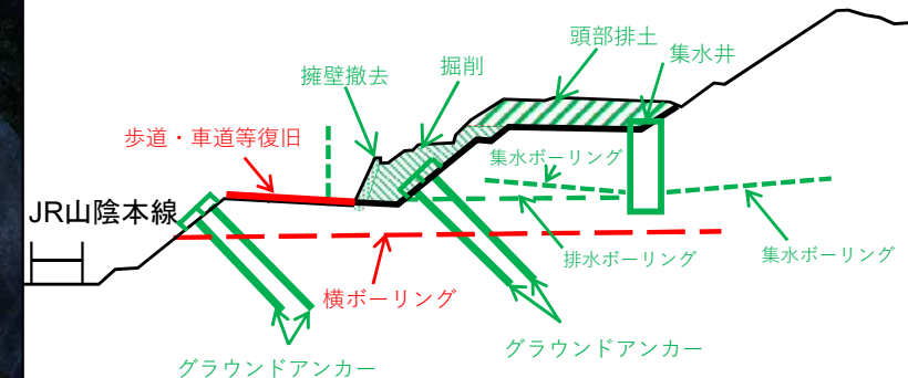
A-A断面
