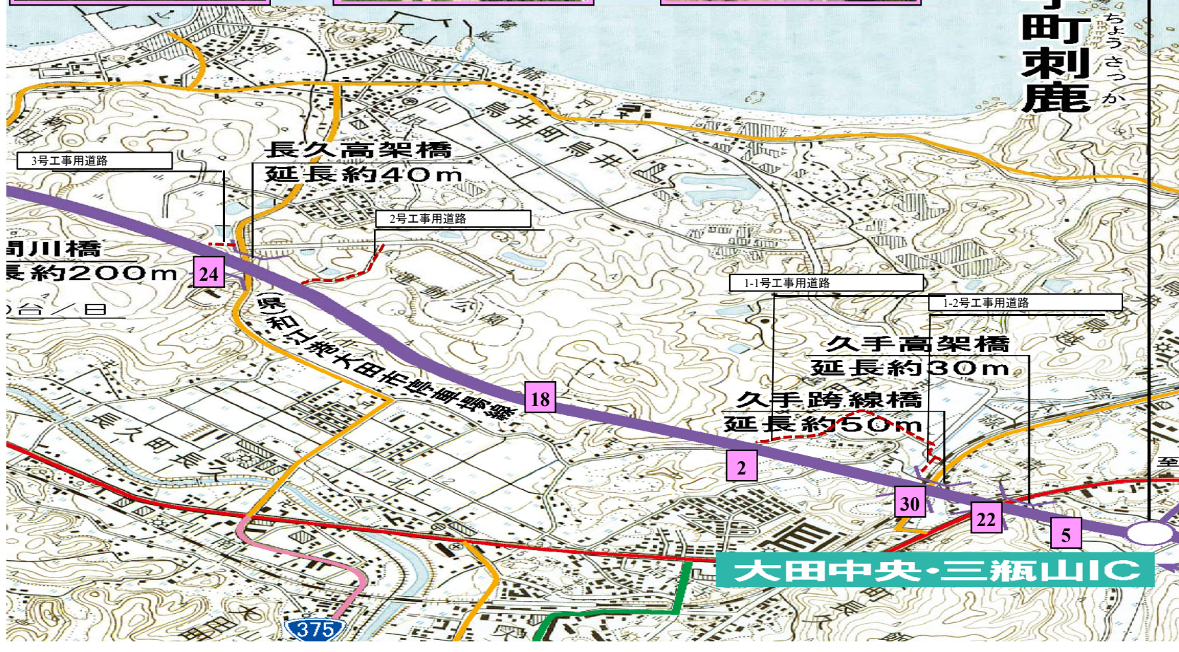
30. 久手跨線橋下部工事 概要：橋梁下部 受注者：松江土建㈱
