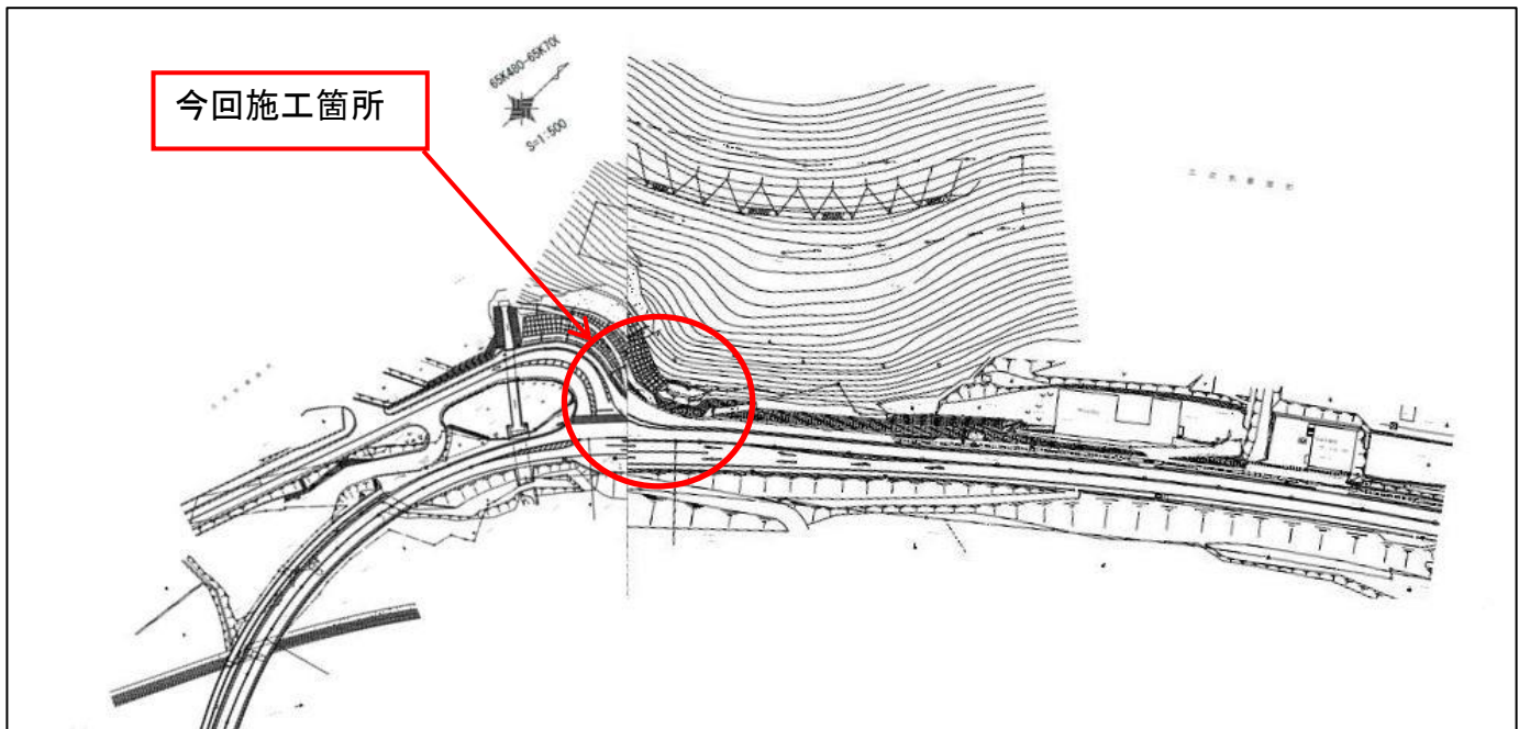
平面図
