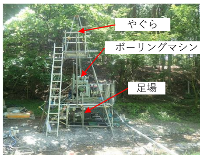
ボーリング調査状況
