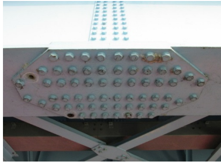
管理橋 継ぎ手部の高力ボルトの脱落
